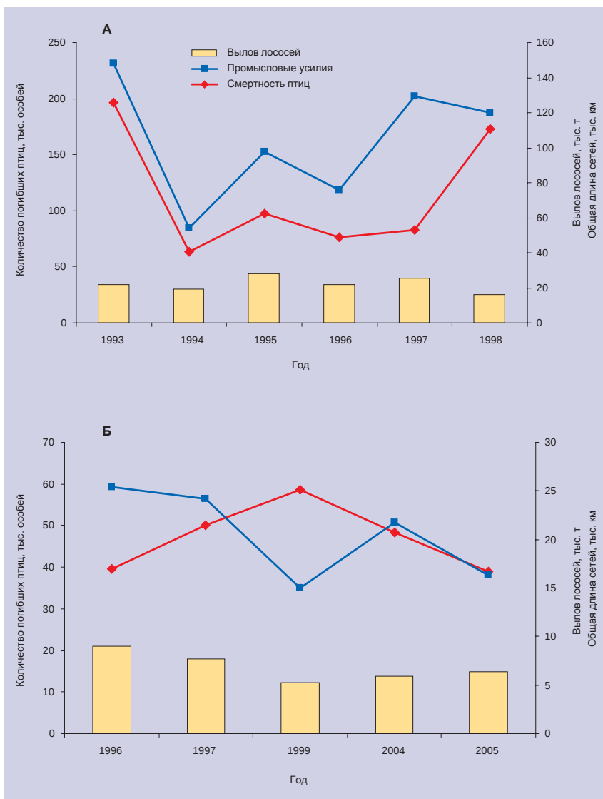
Рис. 89. Оценки смертности морских птиц и характеристики активности (вылов и промысловые усилия) японского (А) и российского (Б) флота в годы мониторинга прилова на дрифтерном промысле лососей в ИЭЗ РФ
