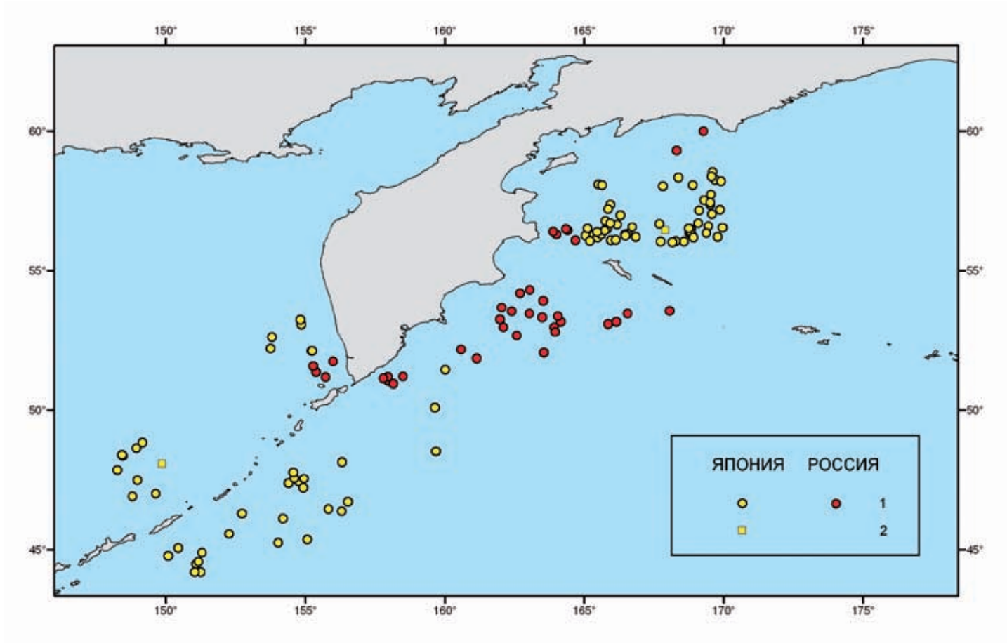
Пункты попадания в сети ушастых тюленей – северного морского котика (1) и сивуча (2) на японском и российском дрейтерном промысле лососей в ИЭЗ РФ
