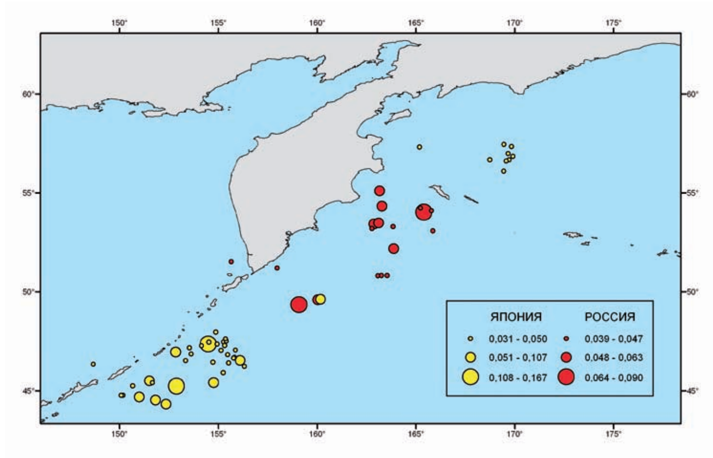
Распределение значений частоты попадания в сети темноспинного альбатроса (количество особей на 1 км сетей) на японском и российском дрейферном промысле лососей в ИЭЗ РФ
