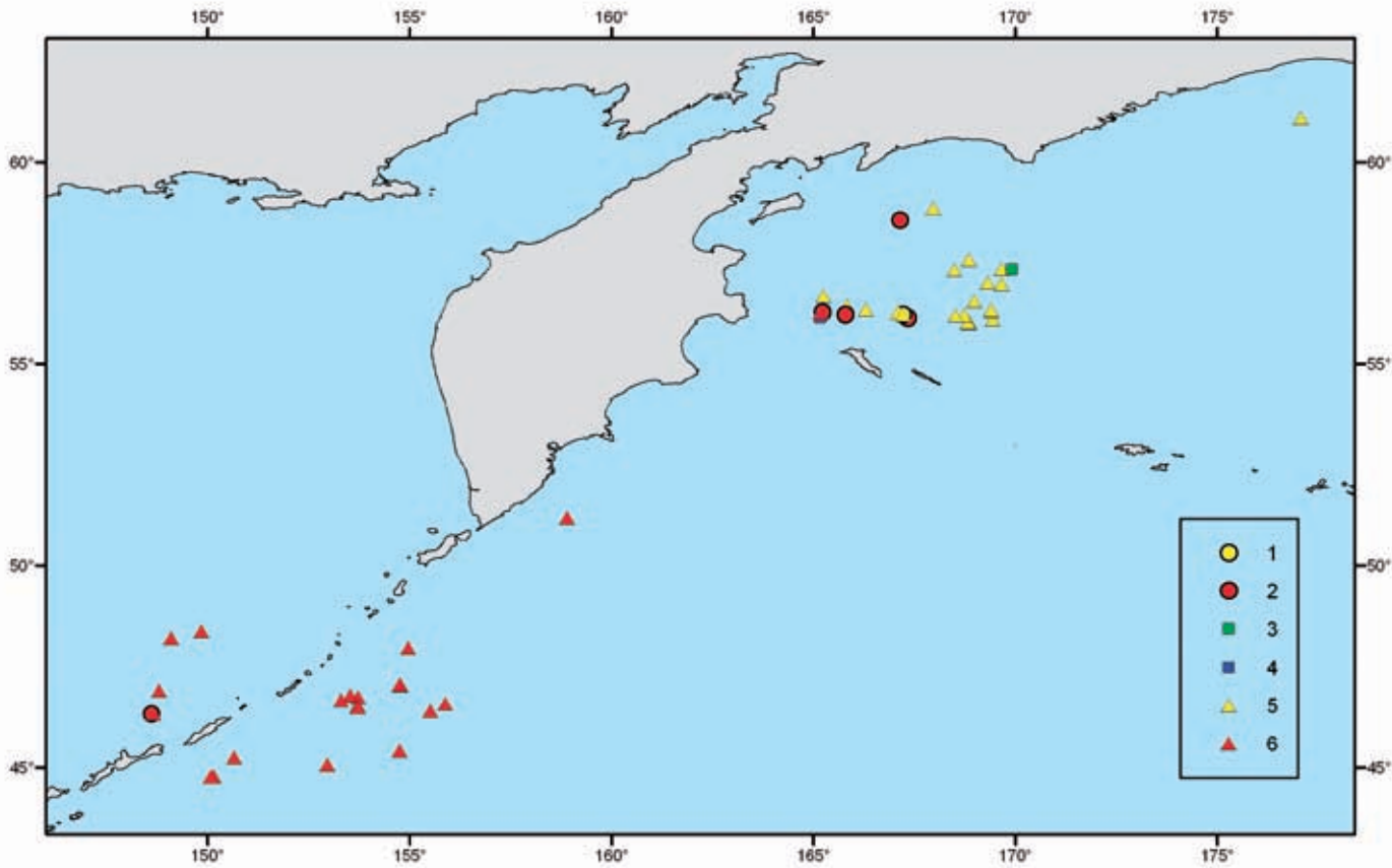
Пункты находок в сетях люрика (1), тихоокеанского чистика (2), пестрого (3), короткоклювого (4) и алеутского (5) пыжиков, тупика-носорога (6) на японском и российском дрейфтерном промысле лососей в ИЭЗ РФ
