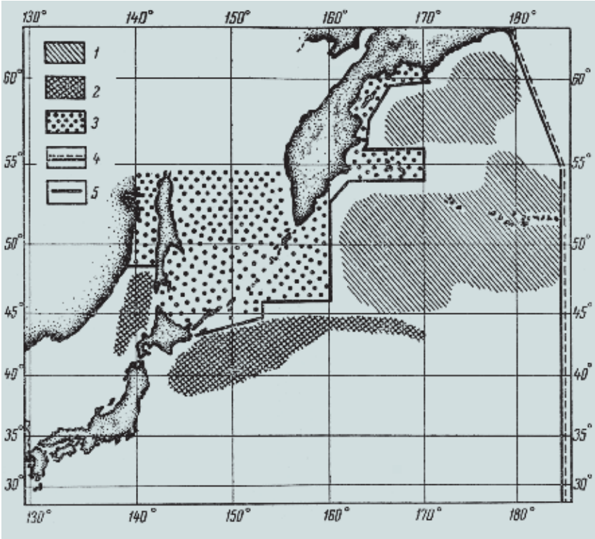
Рис. 14. Районы промысла лососей японским дрейферным флотом после заключения Советско-Японской конвенции 1956 г. (по: Моисеев, 1967): 1 – район лова с судов, базирующихся на плавучие базы; 2 – район лова с судов, базирующихся на порты Японии; 3 – запретный для лова лососей район; 4 – граница района регулирования в соответствии с Советско-Японской рыболовной конвенцией; 5 – граница запретного для лова района
