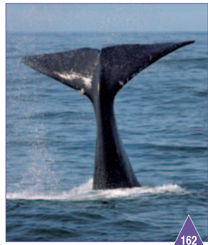
Рис. 162. Гладкий кит; на основании хвостового плавника видны характерные шрамы от запутывания в орудиях рыболовства (Кроноцкий залив, 29 мая 2009 г., фото С. В. Фомина)
