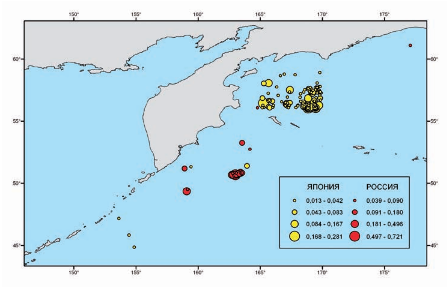
Распределение значений частоты попадания в сети конюги-крошки (количество особей на 1 км сетей) на японском и российском дрейтерном промысле лососей в ИЭЗ РФ
