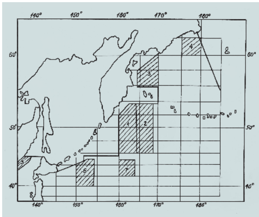
Рис. 17. Меры регулирования японского морского дрифтерного промысла в 1976 г. (по: Вронский, 1980). Сплошная линия — граница конвенционного района. Общая квота вылова — 85 тыс. т. Район 1 — промысел начинается не ранее 26 июня; район 2 — с начала промысла до 20 июня работают не более 3 флотилий; район 3 — работают не более 2 флотилий; район 4 — промысел заканчивается 30 июня; район 5 — запрет промысла до 10 мая; район 6 — с начала промысла до 30 мая работают не более 100 судов; район 7 — с начала промысла до 30 мая работают не более 150 судов
