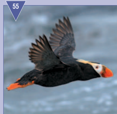
Рис. 50. Толстоклювая кайра Рис. 51. Тонкоклювая кайра Рис. 52. Ипатка Рис. 53. Тихоокеанский чистик Рис. 54. Тупик-носорог Рис. 55. Топорок
