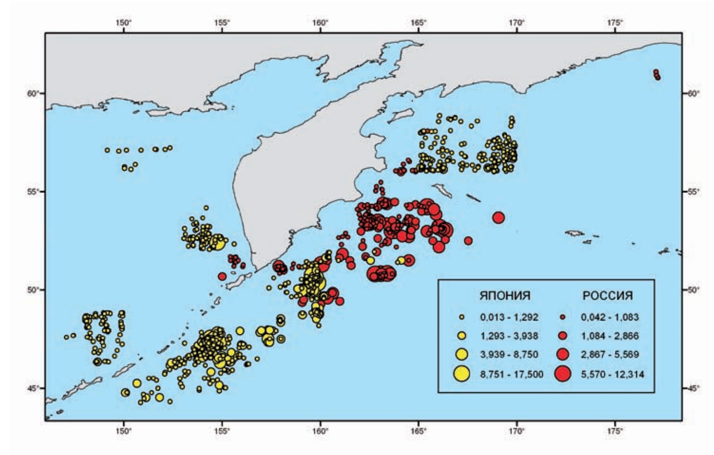
Распределение значений частоты попадания в сети серого и тонкоклювого буревестников (количество особей на 1 км сетей) на японском и российском дрейтерном промысле лососей в ИЭЗ РФ
