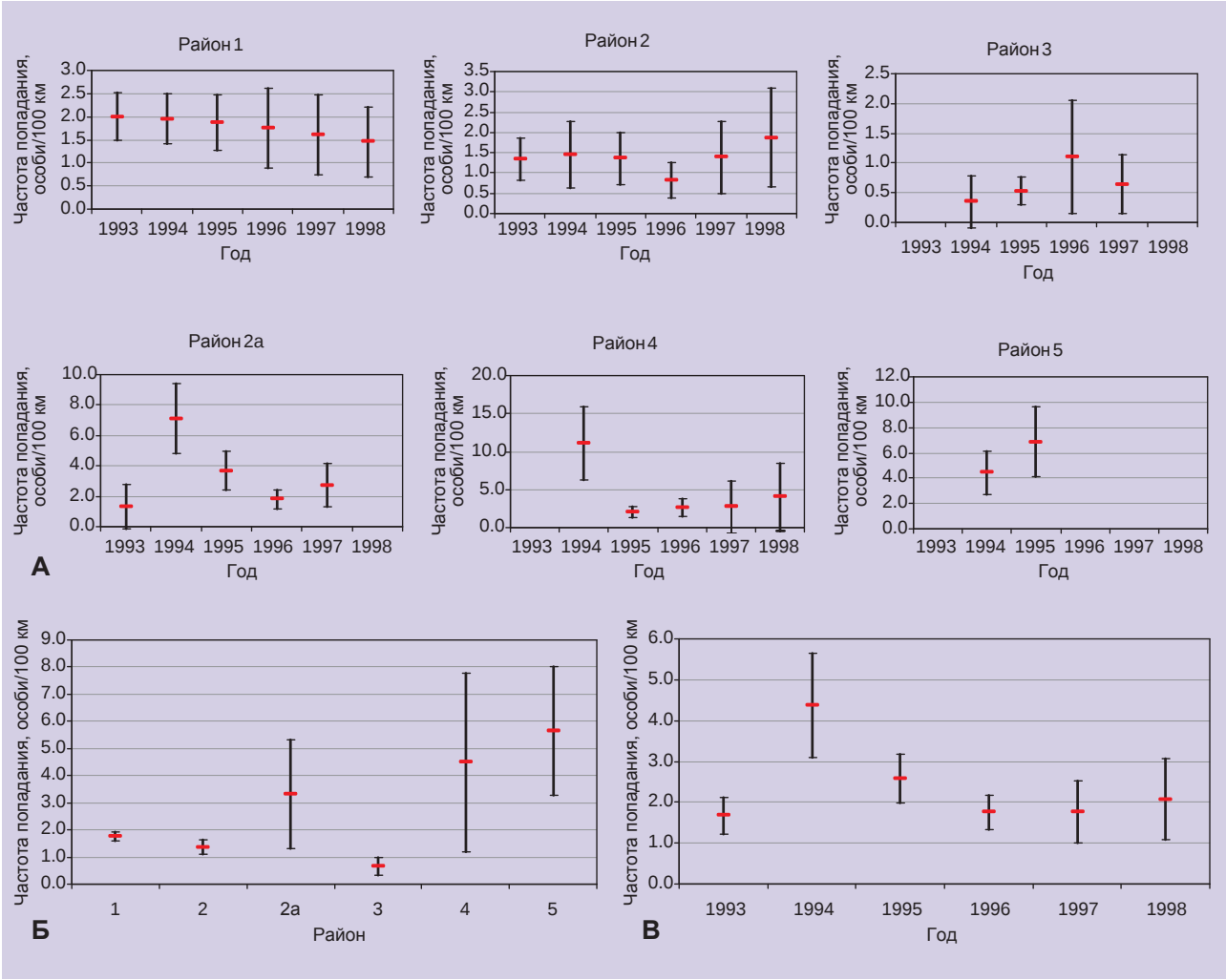
Рис. 111. Частота прилова морских млекопитающих ( M ± 2SD ) на японском дрейферном промысле лососей в ИЭЗ РФ, 1993-1998 гг.: А – по районам и годам; Б – по районам за все годы; В – по годам по всем районам
