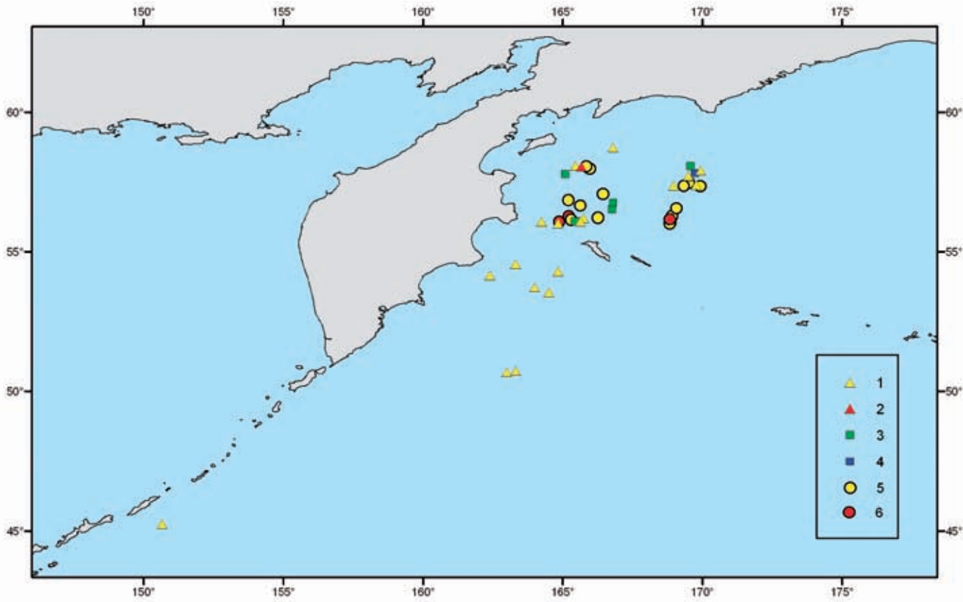
Пункты находок в сетях среднего (1) и длиннохвостого (2) поморников, тихоокеанской чайки (3), бургомистра (4), моевки (5) и красноногой говорушки (6) на японском и российском дрифтерном промысле лососей в ИЭЗ РФ
