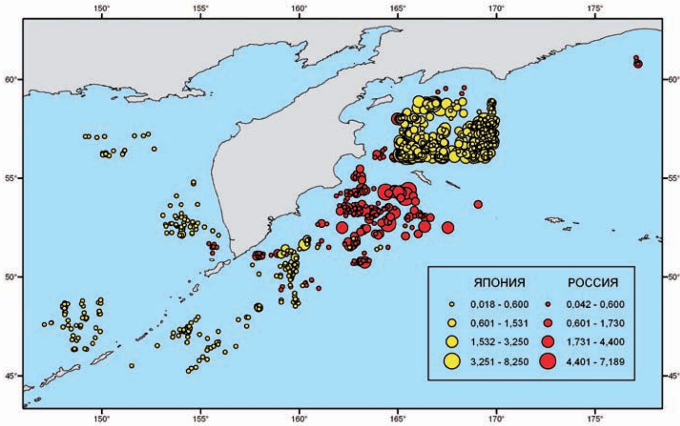
Распределение значений частоты попадания в сети тонкоклювой и толстоклювой кайр (количество особей на 1 км сетей) на японском и российском дрифтерном промысле лососей в ИЭЗ РФ
