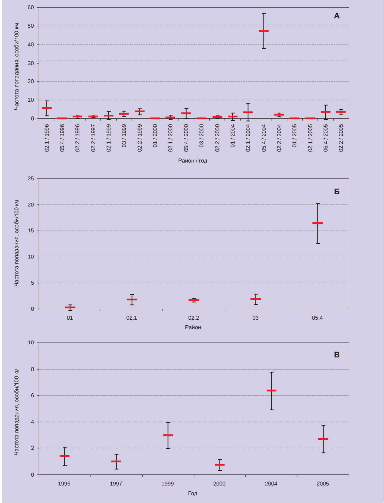
Рис. 117. Частота прилова морских млекопитающих ( M \pm 2SD ) на российском дрейфтерном промысле лососей в ИЭЗ РФ, 1996-2005 гг.: А – по районам и годам; Б – по годам во всех районах; В – по районам за все годы
