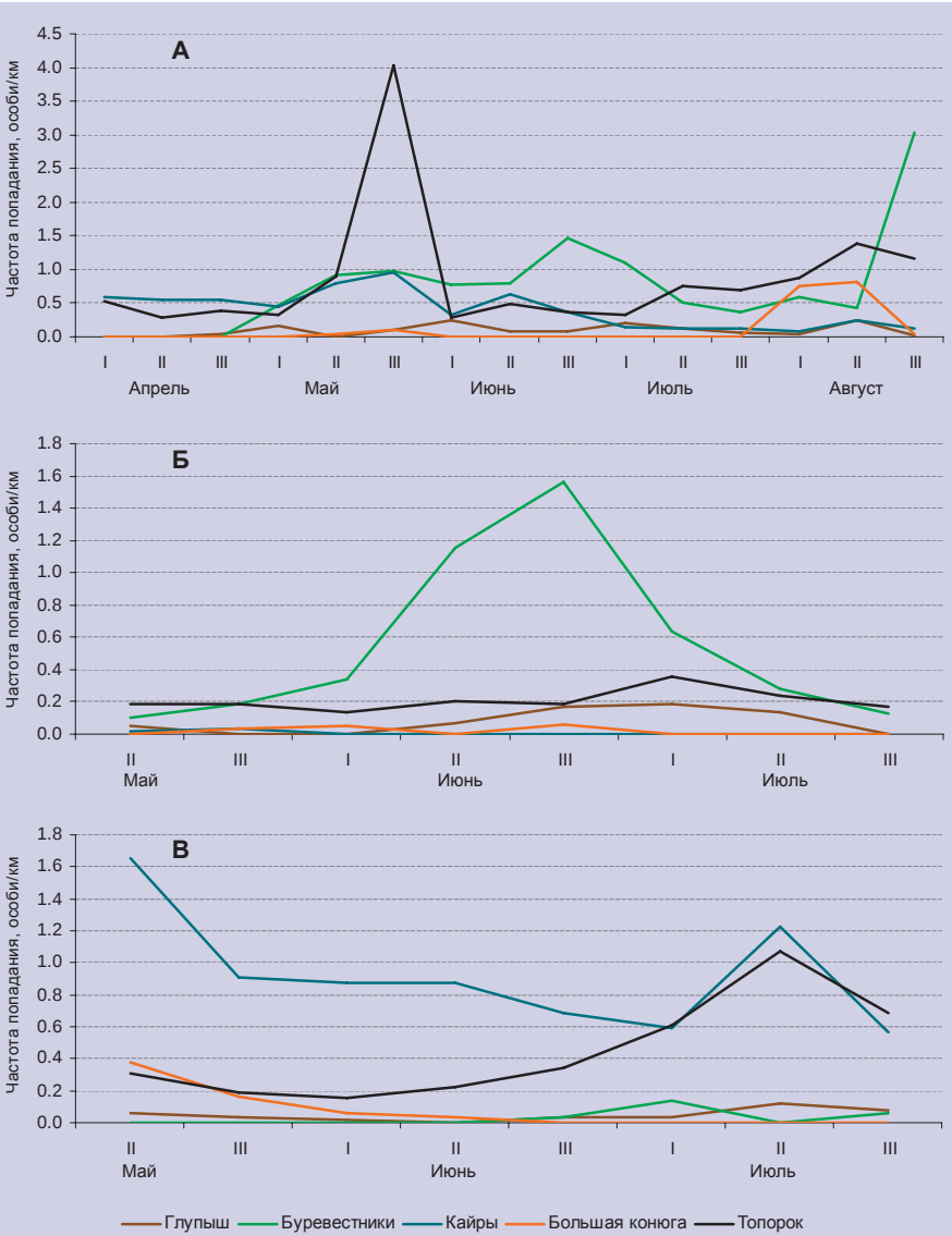
Рис. 81. Динамика частоты попадания морских птиц в сети по декадам промыслового сезона на дрейтерном промысле лососей: А – российский промысел в Петропавловск-Командорской подзоне в 1996-2005 гг.; Б – японский промысел в тихоокеанских водах Курильских о-вов (2-й район) в 1993-1998 гг.; В – японский промысел в Беринговом море (1-й район) в 1993-2001 гг.
