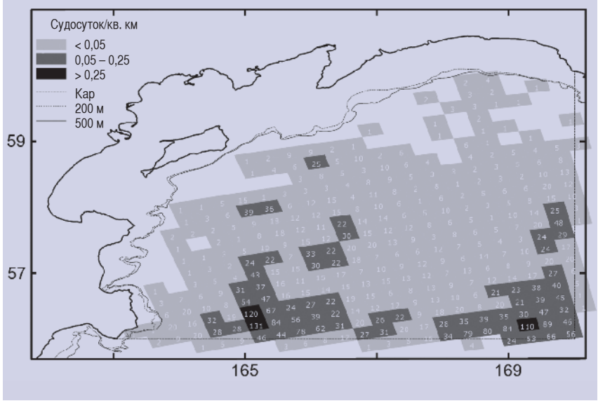
Рис. 94. Схема распределения усилий на дрейфтерном промысле лососей в Карагинской подзоне за 2001-2007 гг. (по: Василец, Терентьев, 2009). Линиями обозначены границы подзоны и изобаты, штриховкой – градации усилий (судосутки на плаву/км 2 ). Цифры внутри отдельных полигонов – общее количество промысловых операций в этом полигоне за весь период
