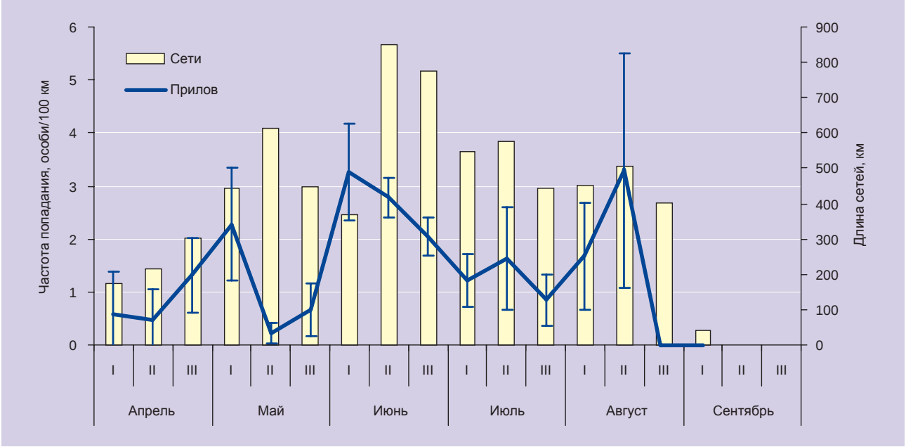
Курильском районе (подзона 05.4). Он превышал расчетную среднюю величину прилова более чем в 20 раз и оказывал существенное влияние на средний показатель частоты попадания зверей в сети не только по годам (2004 г. он был более чем в 3 раза выше) или районам (прилов в районе 05.4 был в 9 раз выше, чем в любом другом районе), но и на объединенную среднюю за все годы и по всем районам. Так, при объединении данных за все годы и по всем районам средняя величина прилова составляла 2,37 \pm 0,35 особей/100 км. При исключении из анализа аномального показателя, средняя величина уменьшалась примерно на 30% и составляла 1,69 \pm 0,30 особей/100 км поднятых сетей (табл. 33).
