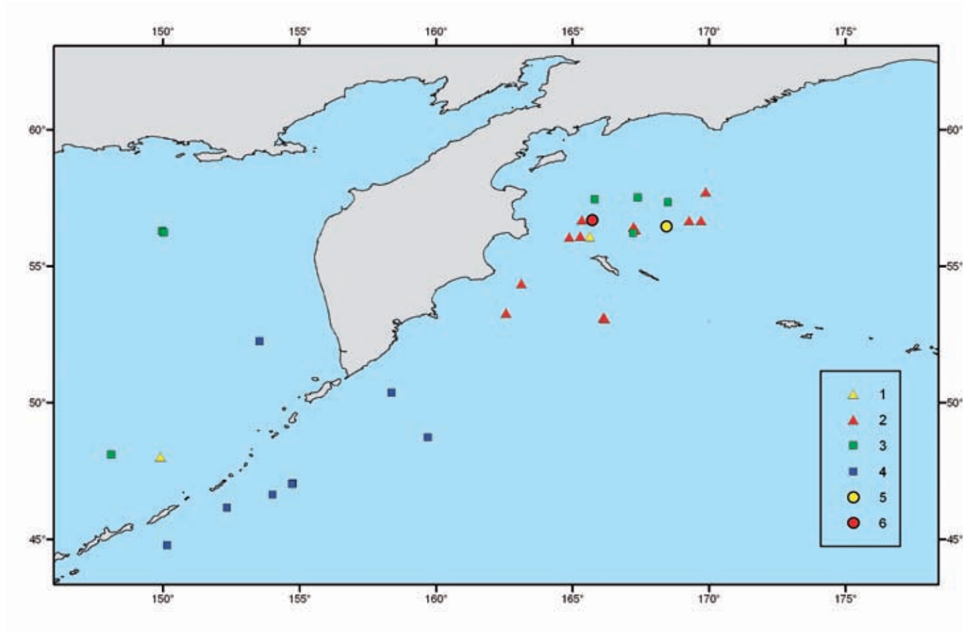
Пункты находок в сетях краснозобой (1), чернозобой (2) и белоклювой (3) гагар, северной качурки (4), берингова (5) и краснолицего (6) бакланов на японском и российском дрейфтерном промысле лососей в ИЭЗ РФ
