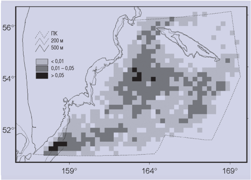
Рис. 95. Схема распределения усилий на дрейфтерном промысле лососей в Петропавловско-Командорской подзоне за 2001-2006 гг. (по: Василец, Терентьев, 2008). Линиями обозначены границы подзоны и изобаты, штриховкой – градации усилий (судосутки на плаву/км 2 )
