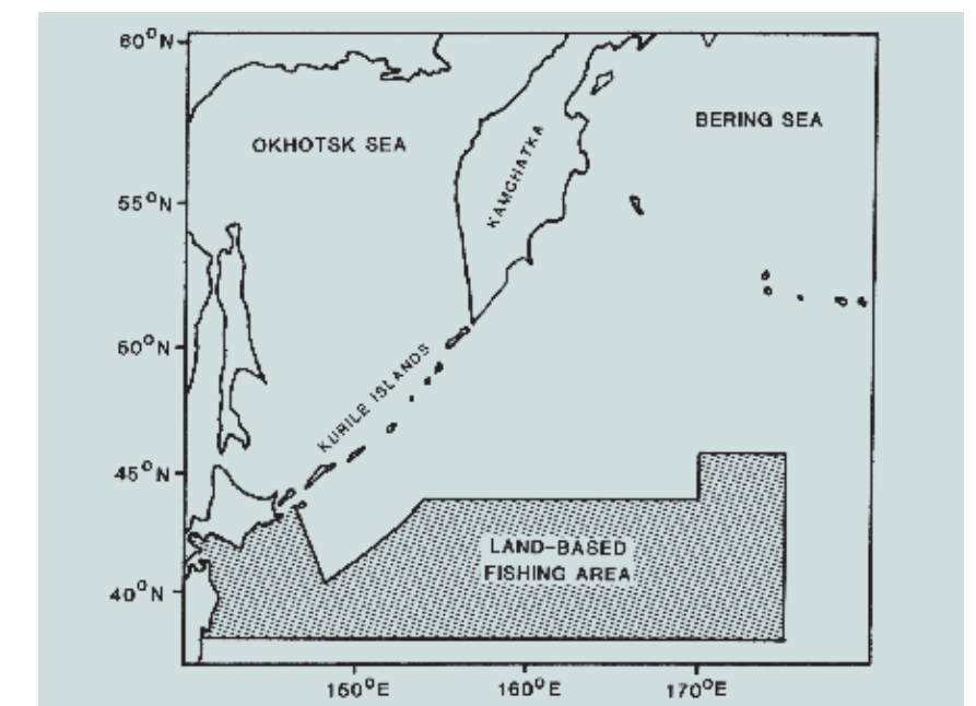
Рис. 22. Район промысла лососей японскими судами, базирующимися на порты Японии, после введения 200-мильных экономических зон (по: DeGange, Day, 1991)
