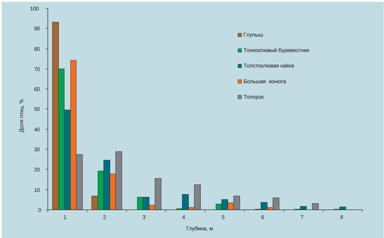
Рис. 169. Распределение массовых видов морских птиц по высоте сетного полотна на японском дрифтерном промысле лососей в ИЗЗ РФ, 1996-1997 гг.
