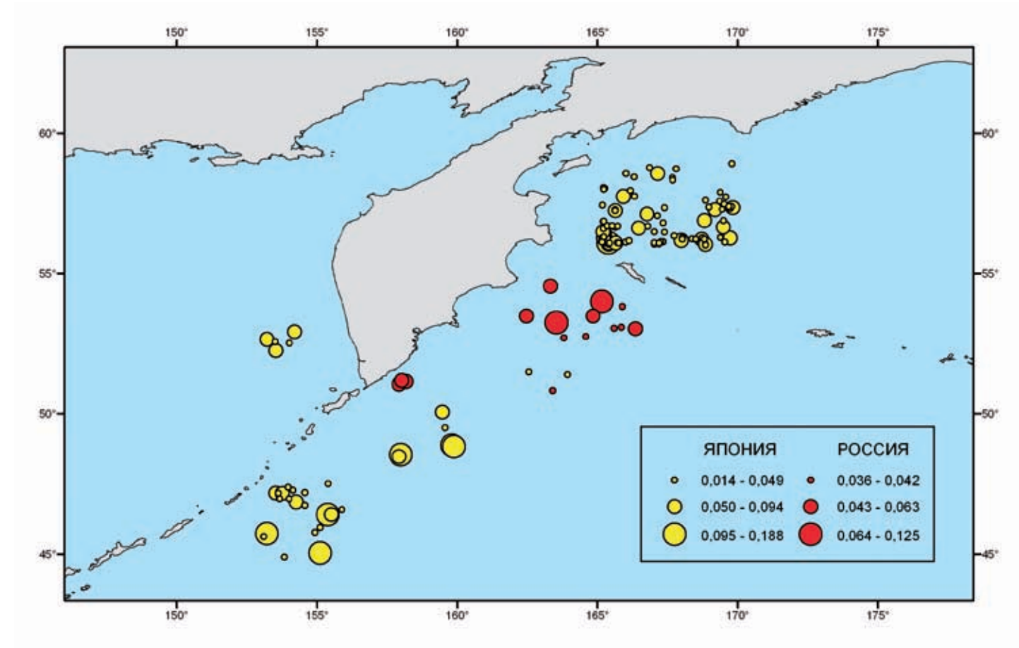
Распределение значений частоты попадания в сети белобрюшки (количество особей на 1 км сетей) на японском и российском дрейтерном промысле лососей в ИЭЗ РФ
