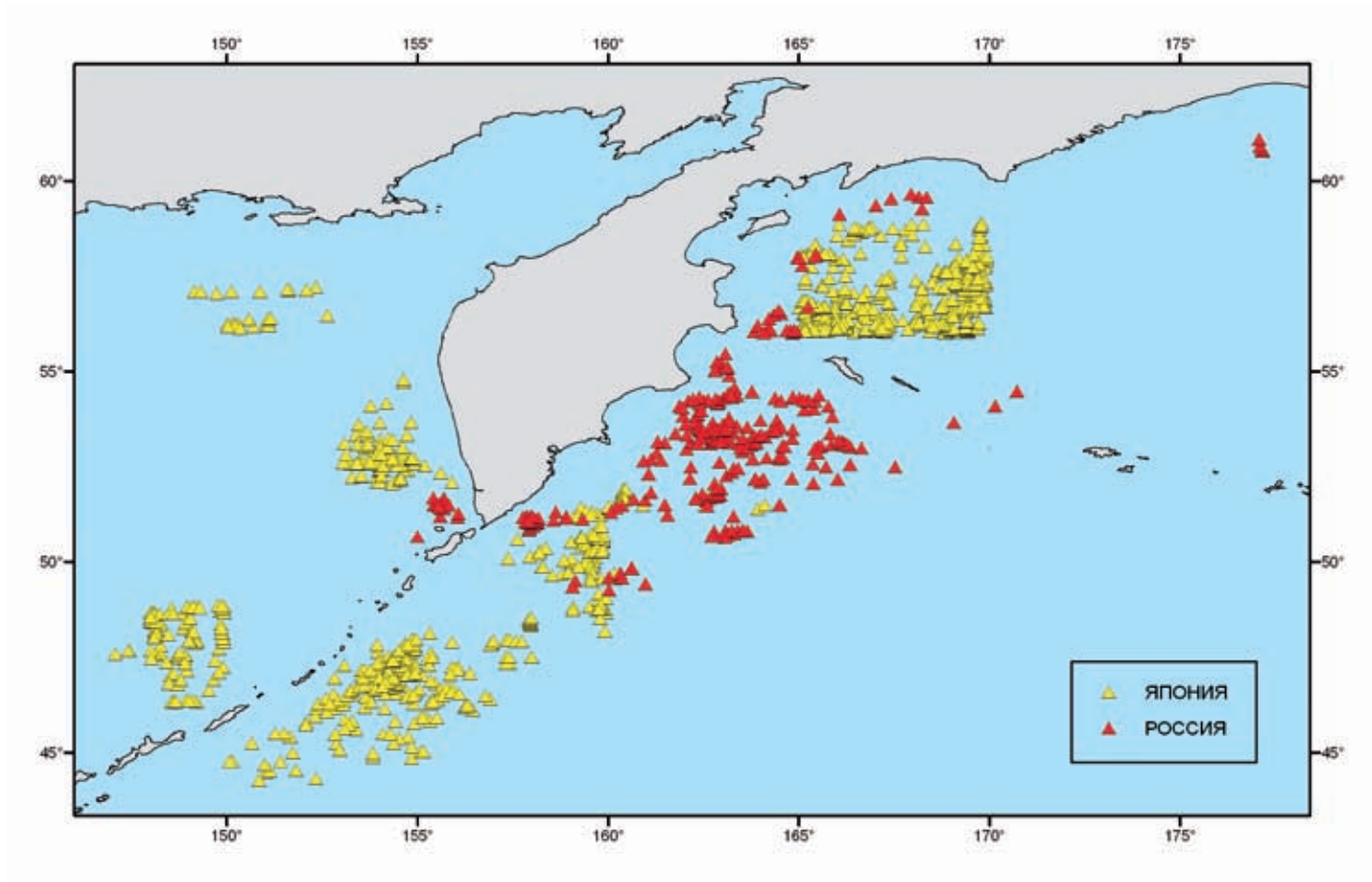
Распределение контрольных сетедрейфов, на которых проводилось определение видового состава погибших в сетях птиц, на японском (1993-2001 гг.) и российском (1996-2005 гг.) дрейферном промысле лососей в ИЭЗ РФ
