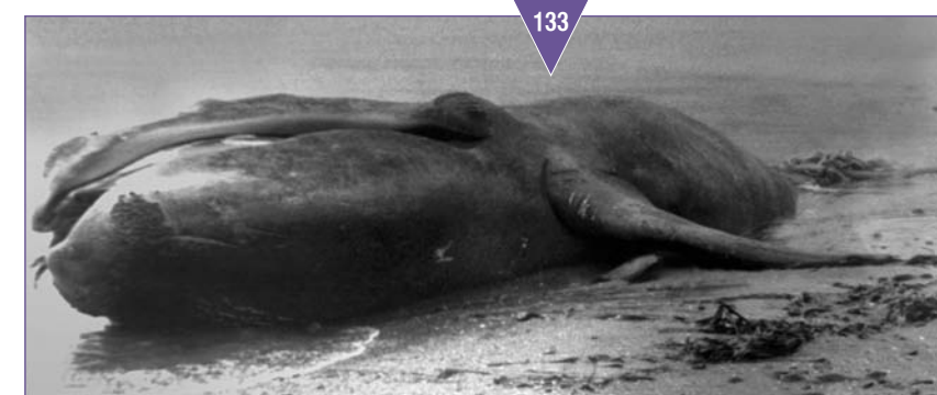
Рис. 133. Погибший гладкий кит с фрагментом дрейфтерной сети на хвостовом стебле (м. Лопатка, Камчатка, октябрь 1989 г., фото С. И. Корнева)
