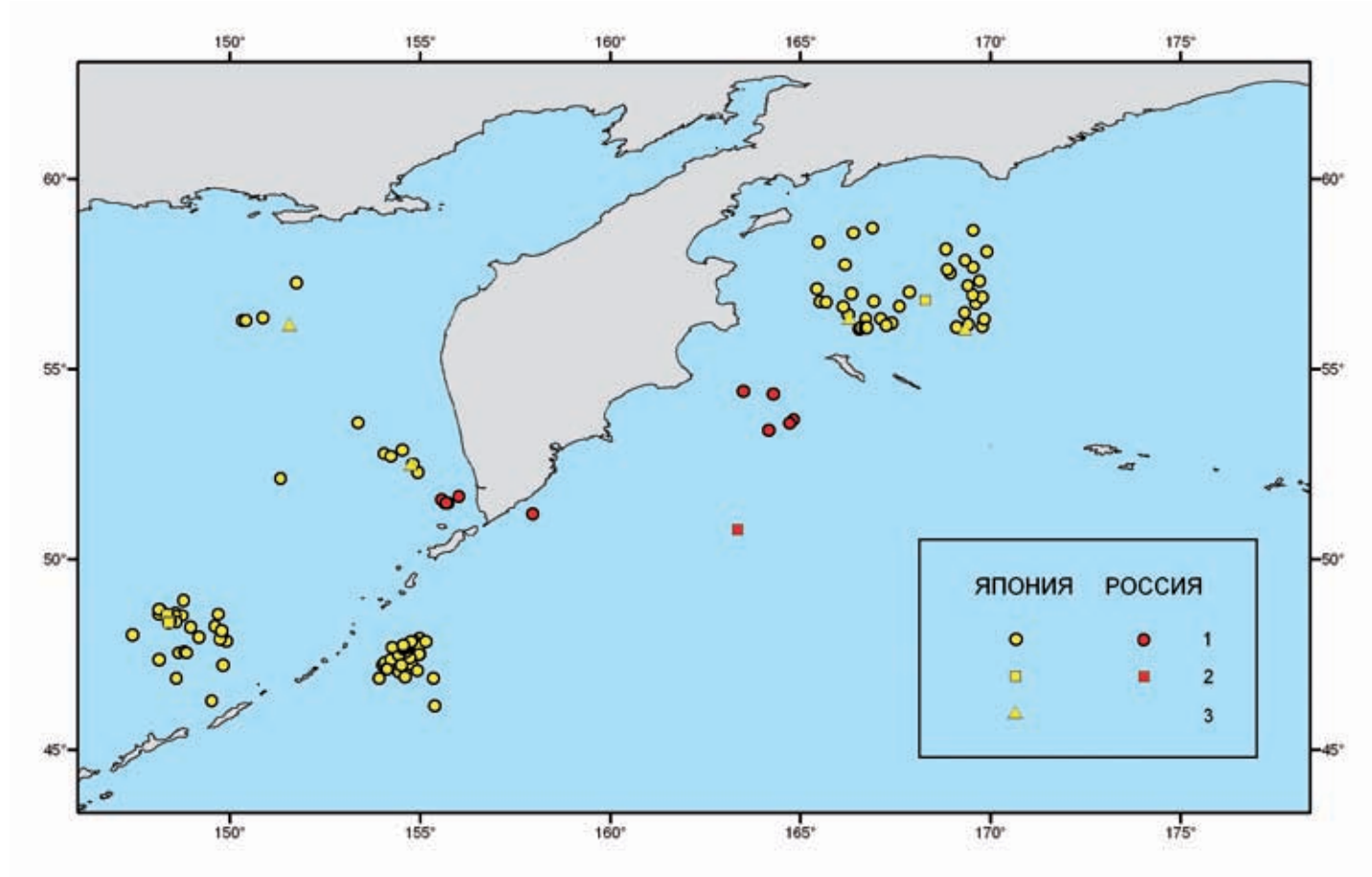
Пункты попадания в сети настоящих тюленей – крылатки (1), ларги (2) и кольчатой нерпы (3) на японском и российском дрейтерном промысле лососей в ИЭЗ РФ
