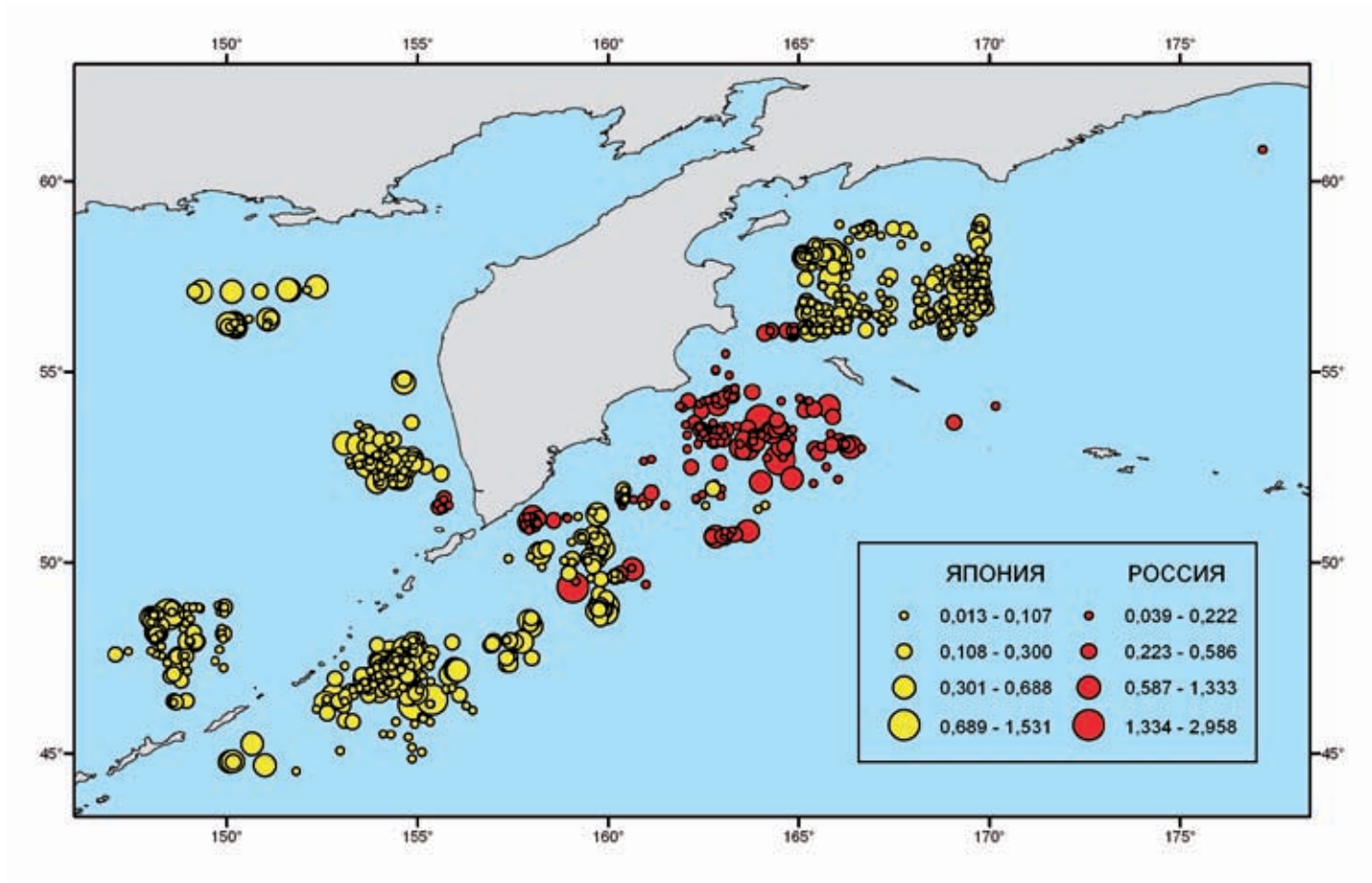
Распределение значений частоты попадания в сети глупыша (количество особей на 1 км сетей) на японском и российском дрейтерном промысле лососей в ИЭЗ РФ
