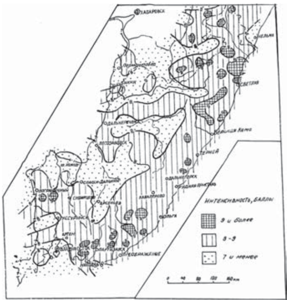
Рис. 2. Схема сейсморайонирования по палеосейсмогеологическим данным
