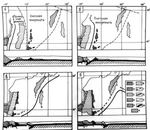
Рис. 19. Карта палеогеографической эволюции структур фундамента ландшафтов тихоокеанской зоны Востока России
