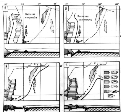
Рис. 7. Карта положения и эволюции основных палеоструктур
