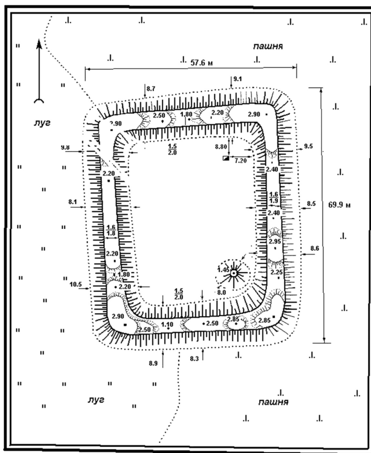
Рис. 40. План городища Уборка-Долинное (Усть-Павловка) (Съемка О.Ю. Тарасова)
