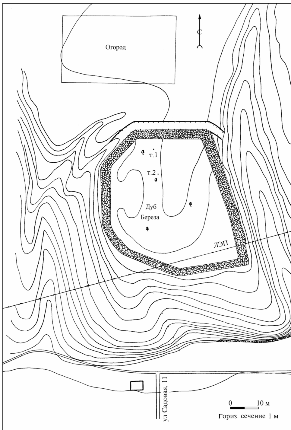
Рис. 54. План городища Горнореченское-3
