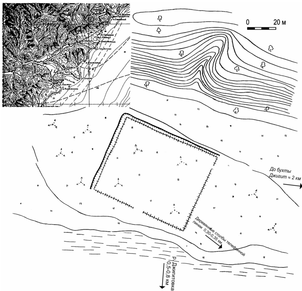
Рис. 77. План городища Красное Озеро
