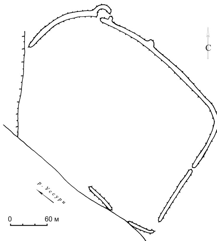
Рис. 38. План городища Кокшаровка-II (съемка В.И. Дьякова)
