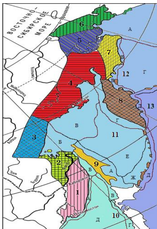
Рис. 9. Карта ландшафтных областей, провинций работ «Агроландшафтного сектора» ДВФУ (Старожилов, 2021. Фрагмент карты районирования нооландшафтосферы планеты Земля). Области пояса: 1. Сихотэ-Алинская; 2. Нижнеамурская; 3. Прихотская; 4. Колымская; 5. Анадырская; 6. Чукотская; 7. Корякская; 8. Камчатско-Курильская; 9. Сахалинская; 10. Японская; 11. Охотская; 12. Беринговая; 13. Тихоокеанская; Провинции областей окраинных морей: японской (10): шельфовые – А. Западная японская; Б. Северояпонская; В. Восточносахалинская; Г. Восточная японская; морская: Д. Центральная японская; охотской (11): шельфовые: А. Запдноохотскосахалинская; Б. Запдноохотская; В. Колымскоохотская; Г. Охотскокамчатская; Д. Камчатскокурильская; Ж. Охотскокурильская; морская: Е. Центральная охотская; беринговой (12): шельфовые: А. Командорскоберинговая; Б. Корякскоберинговая; В. Камчатскоберинговая; Д. Тихоокеанскокурильскокамчатская; морская: Г. Центральноберингова
