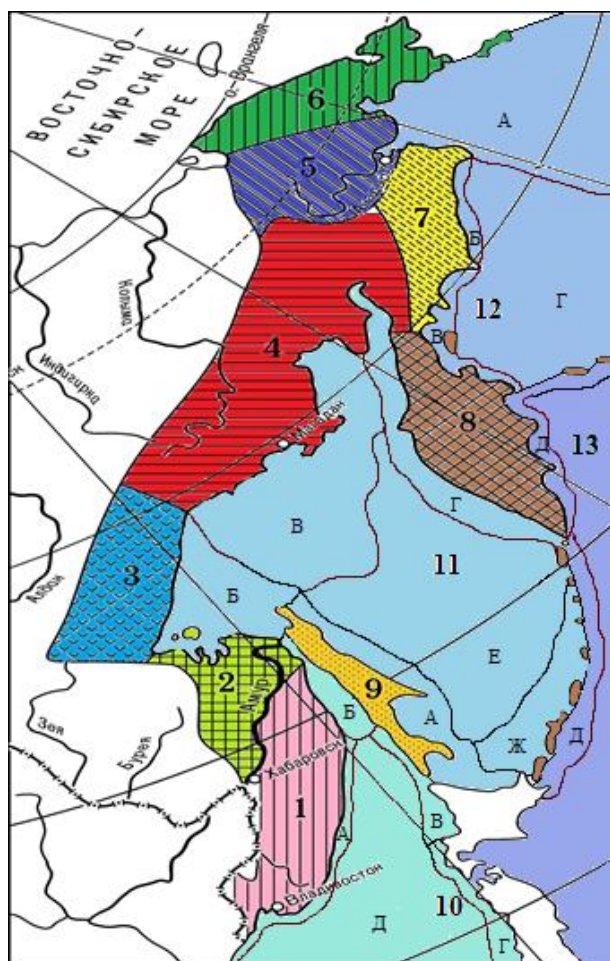
Рис. 20. Карта районирования морского звена Тихоокеанского ландшафтного пояса России. (Старожилов, 2021. Фрагмент карты районирования ноо ландшафтосферы планеты Земля) Области пояса:
