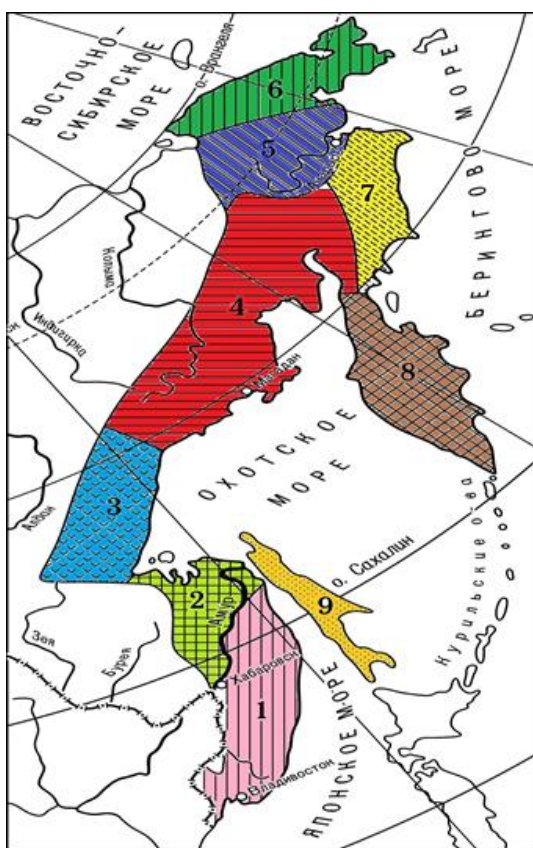
Рис. 14. Карта притихоокеанских орогенных ландшафтных областей Востока России. Области: 1. Сихотэ-Алинская; 2. Нижнеамурская; 3. Приохотская; 4. Колымская; 5. Анадырская; 6. Чукотская; 7. Корякская; 8. Камчатско-Курильская; 9. Сахалинская
