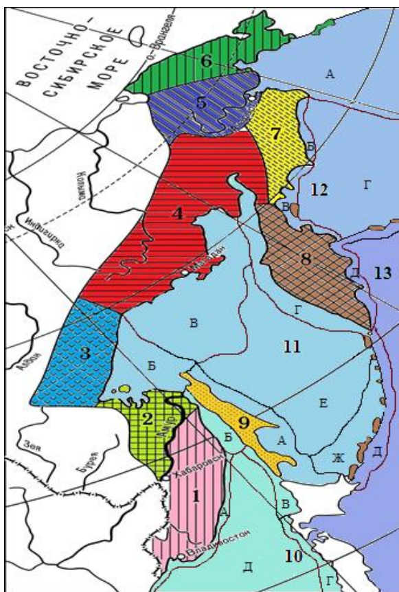
Рис. 1. Карта Тихоокеанского ландшафтного пояса России, его областей, провинций (Старожилов, 2021. Фрагмент карты районирования нооландшафтосферы планеты Земля). Области пояса: 1. Сихотэ-Алинская; 2. Нижнеамурская; 3. Приохотская; 4. Колымская; 5. Анадырская; 6. Чукотская; 7. Корякская; 8. Камчатско-Курильская; 9. Сахалинская; 10. Японская; 11. Охотская; 12. Беринговая. 13. Тихоокеанская; Провинции областей окраинных морей: японской (10): шельфовые – А. Западная японская; Б. Северояпонская; В. Востоочносахалинская; Г. Восточная японская; морская: Д. Центральная японская; охотской (11): шельфовые: А. Западноохотскосахалинская; Б. Западноохотская; В. Колымскоохотская; Г. Охотскокамчатская; Д. Камчатскокурильская; Ж. Охотскокурильская; морская: Е. Центральная охотская; беринговой (12): шельфовые: А. Командорскоберинговая; Б. Корякскоберинговая; В. Камчатскоберинговая; Д. Тихоокеанскокурильскокамчатская; морская: Г. Центральная беринговая
