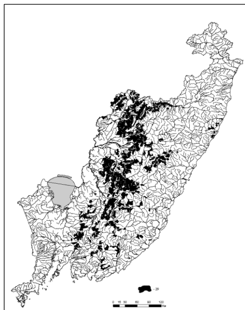
Рис. 11. Распространенность низогорных широколиственно-кедровых лесных ландшафтов горно-лесного смешанно-широколиственного пояса
