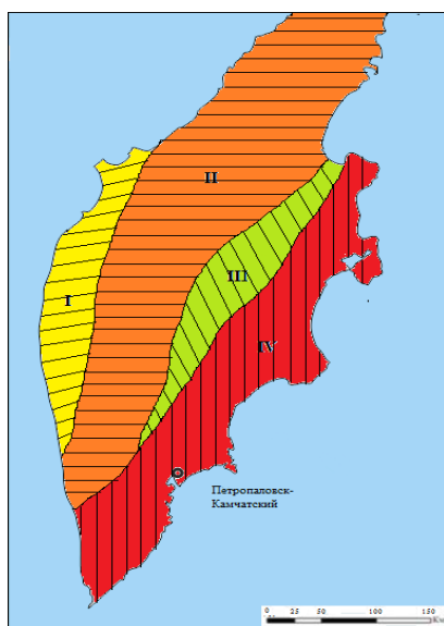
Рис. 17. Ландшафтные провинции полуострова Камчатка: I – Западно-Камчатская; II – Срединно-Камчатская; III – Центрально-Камчатская; IV – Восточно-Камчатская
