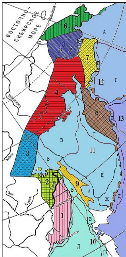
Рис. 10. Карта областей, провинций Тихоокеанского ландшафтного пояса России (Старожилов, 2021.). Области пояса: 1. Сихотэ-Алинская; 2. Нижнеамурская; 3. Приохотская; 4. Колымская; 5. Анадырская; 6. Чукотская; 7. Корякская; 8. Камчатско-Курильская; 9. Сахалинская; 10. Японская; 11. Охотская; 12. Беринговая. 13. Тихоокеанская; Провинции областей окраинных морей: японской (10): шельфовые – А. Западнояпонская; Б. Северояпонская; В. Восточносахалинская; Г. Восточнояпонская; морская: Д. Центральная японская; охотской (11): шельфовые: А. Западноохотско-сахалинская; Б. Западноохотская; В. Колымскоохотская; Г. Охотскокамчатская; Д. Камчатскокурильская; Ж. Охотскокурильская; морская: Е. Центральная охотская; беринговой (12): шельфовые: А. Командорскоберинговая; Б. Корякскоберинговая; В. Камчатскоберинговая; Д. Тихоокеанскокурильскокамчатская; морская: Г. Центральнберинговая
