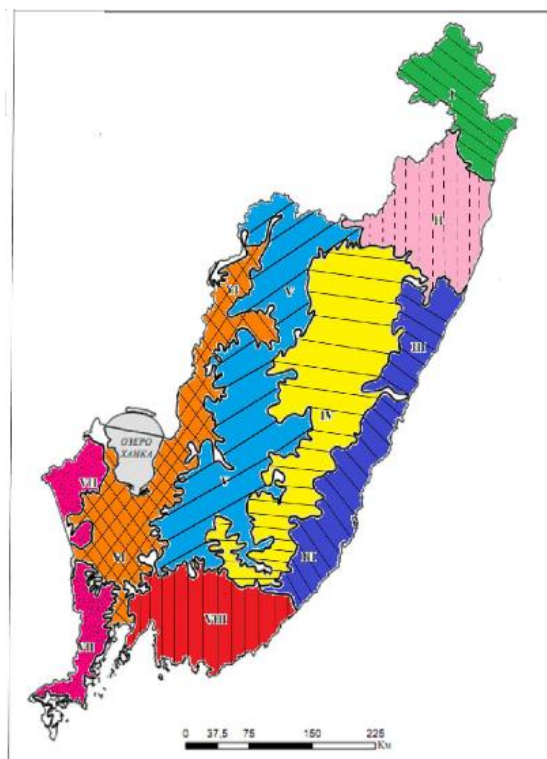
Рис. 15. Ландшафтные провинции Сихотэ-Алинской ландшафтной области:
