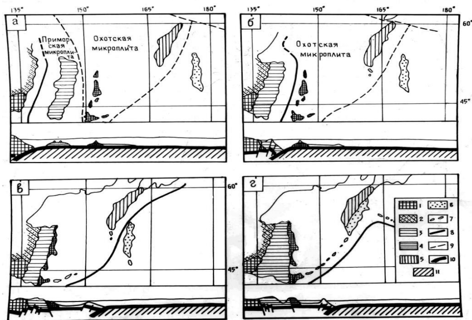
Рис. 27. Карта результатов палеорекострукции фундамента ландшафтов Востока России: 1 – Ханкайский массив. 2 – пассивная палеоокраина Бикино-Баджалло-Нижнеамурской зоны. 3 – Приморское палеоплато Приморской микроплиты с атоллами и рифовыми постройками на вершинах гор. 4 – Хоккайдо-Сахалинский палеохребет юго-западной части Охотской микроплиты с атоллами и рифовыми постройками на вершинах гор. 5 – Западно-Камчатское поднятие. 6 – Восточно-Камчатское поднятие. 7 – современная вулканическая дуга. 8 – сейсмофокальная зона. 9 – предполагаемые границы микроплит. 10 – океаническая кора. 11 – мантия. а, б, в, г – положение палеоструктур в: а – домеловое время, б – бериасе, в – валанжин-датское время, г – в палеоцен-эоцене
