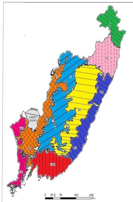
Рис. 24. Пример карты районирования Ландшафтные провинции Приморского края: I – Самаргинская, II – Северо-Сихотэ-Алинская, III – Восточно-Сихотэ-Алинская, IV – Центрально-Сихотэ-Алинская, V – Западно-Сихотэ-Алинская, VI – Западно-Приморская равнина, VII – Восточно-Маньчжурская, VIII – Южно-Приморская
