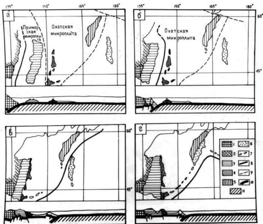
Рис. 19. Карта палеогеографической эволюции структур фундамента ландшафтов тихоокеанской зоны Востока России 1 – Ханкайский массив. 2 – пассивная палеоокраина Бикино-Баджало-Нижнеамурской зоны. 3 – Приморское палеоплато Приморской микроплиты с атоллами и рифовыми постройками на вершинах гор. 4 – Хоккайдо-Сахалинский палеохребет юго-западной части Охотской микроплиты с атоллами и рифовыми постройками на вершинах гор. 5 – Западно-Камчатское поднятие. 6 – Восточно-Камчатское поднятие. 7 – современная вулканическая дуга. 8 – сейсмофокальная зона. 9 – предполагаемые границы микроплит. 10 – океаническая кора. 11 – мантия в океане. а, б, в, з – положение палеоструктур в: а – домеловое время, б – бериасе, в – валанжин-датское время, з – в палеоцен-эоцене
