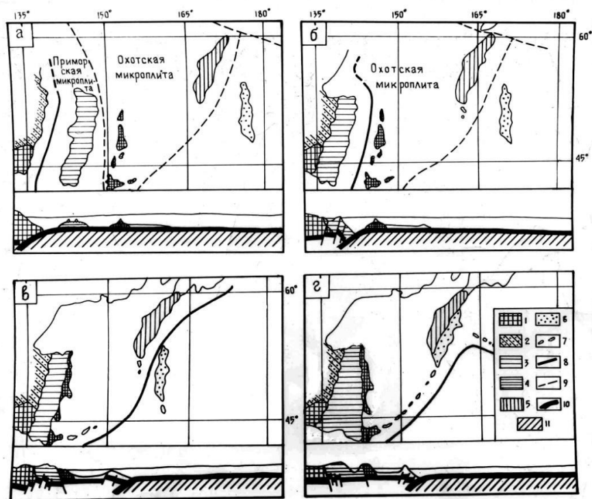
Рис. 13. Схема эволюции фундамента ландшафтов геосистемы Восток России – Тихий океан.
