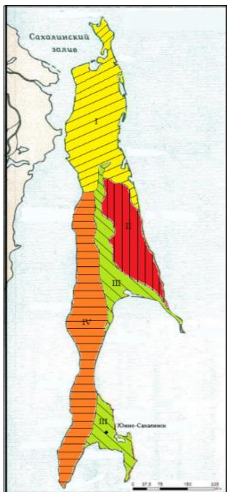
Рис.16. Ландшафтные провинции острова Сахалин:
