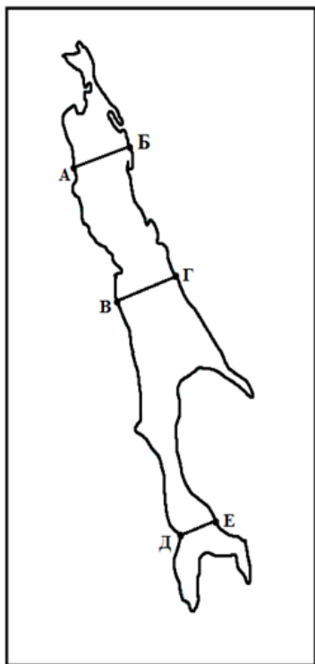
Рис. 22. Профили, проложенные по о. Сахалин
