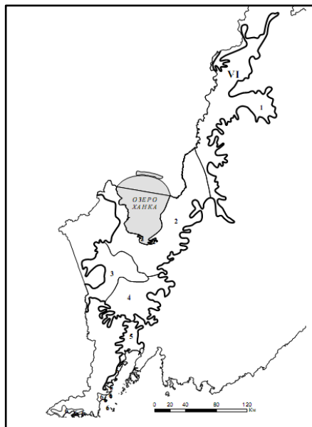
Рис. 12. Пространственное положение Приханкайского ландшафтного округа (2) (Уссури-Ханкайская провинция VI)
