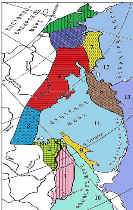
Рис. 18. Карта морских и континентальных ландшафтных областей геосистемы Восток России – Тихий океан (Старожилов, 2018) Области: 1. Сихотэ-Алинская; 2. Нижнеамурская; 3. Приохотская; 4. Колымская; 5. Анадырская; 6. Чукотская; 7. Корякская; 8. Камчатско-Курильская; 9. Сахалинская; 10. Японская; 11. Охотская; 12. Беринговая. 13. Тихоокеанская
