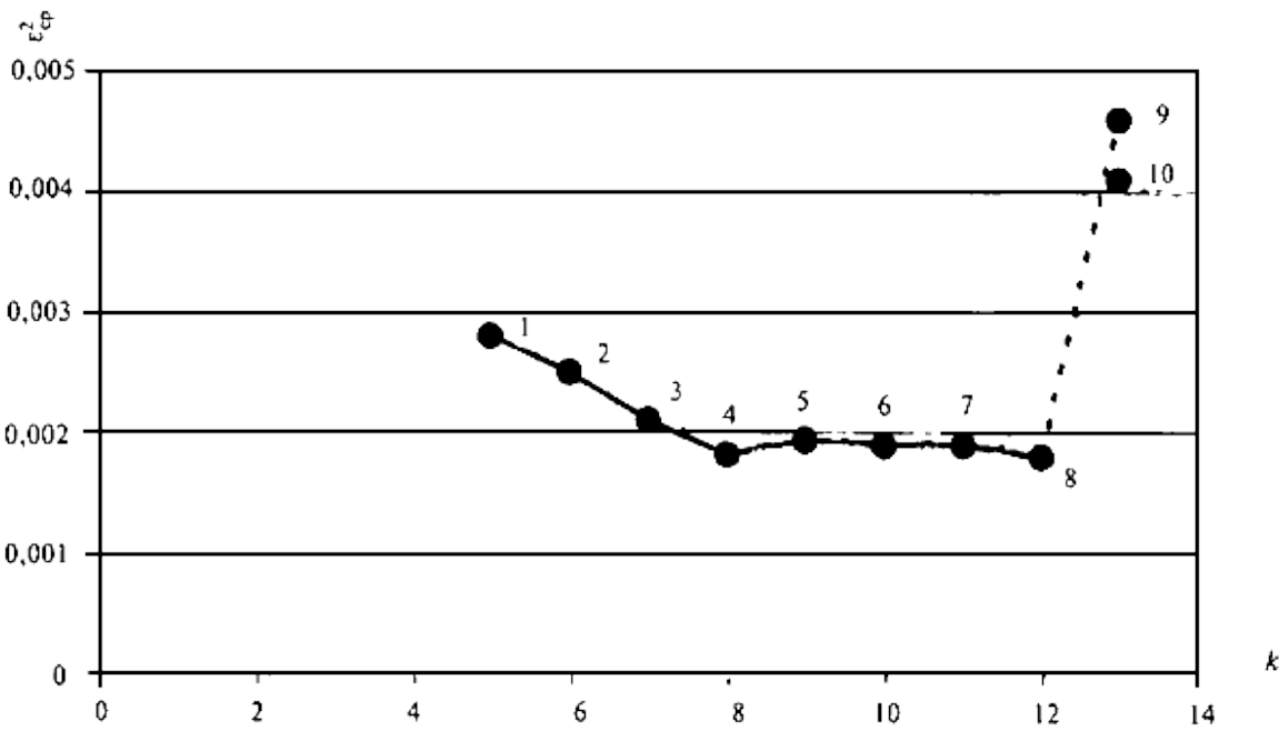
Рисунок А.3 - График зависимости дисперсии параметров объединенной совокупности от числа совместно анализируемых постов Результаты расчета погрешностей определения коэффициента вариации приведены в таблице А.3.
