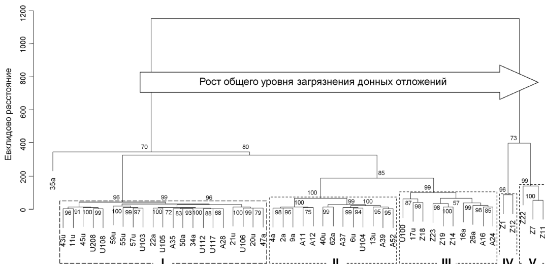
Рис. 4. Дендрограмма сходства станций, опробованных в зал. Петра Великого, полученная методом Уорда (вариант D2, метрика — евклидово расстояние) с несмещенными оценками бутстреп-вероятностей появления узла (цифры в узлах дендрограммы); рамками отмечены выделяемые группы (узлы с вероятностью появления > 95 %)
