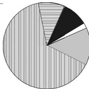
Рис. 3.15. Среднее соотношение трофических групп в сообществе с доминированием собирающих детритофагов. По А.П.Кузнецову (1980). Обозначения как на рис. 3.8.
