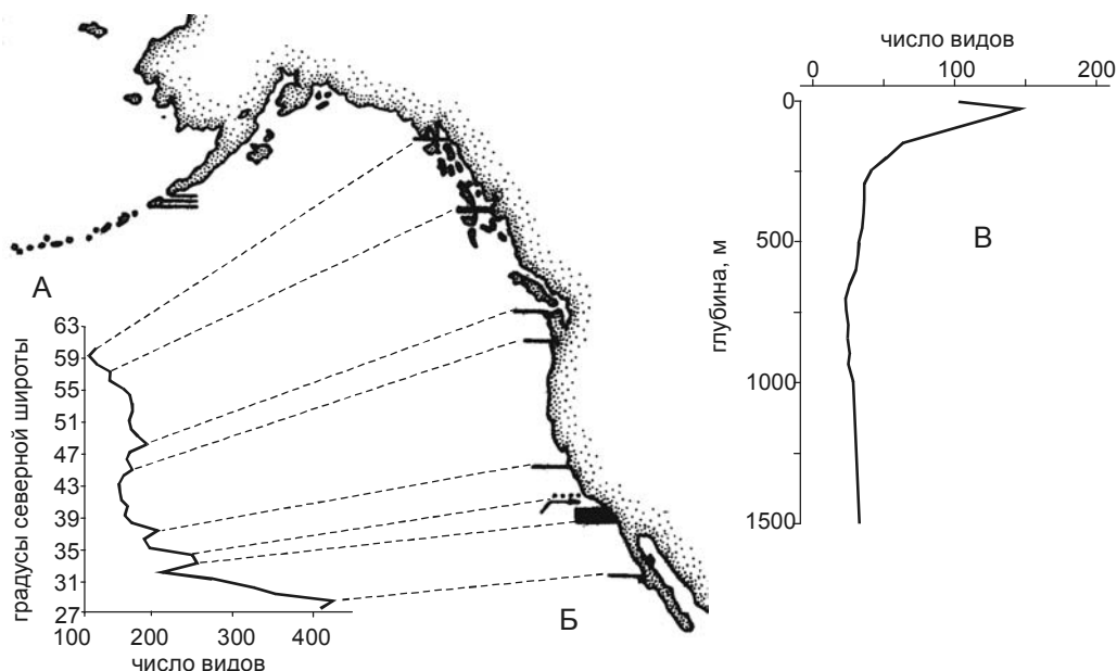
Рис. 5.16. Биотические разрезы.
