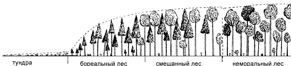
Рис. 5.25. Часть градиента экотона тундра – тропики. По Уиттекеру (1980).
