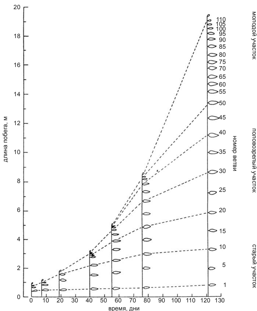
Рис. 3.34. Развитие побега Macrocytis . Показаны не все ветви. По North (1979).
