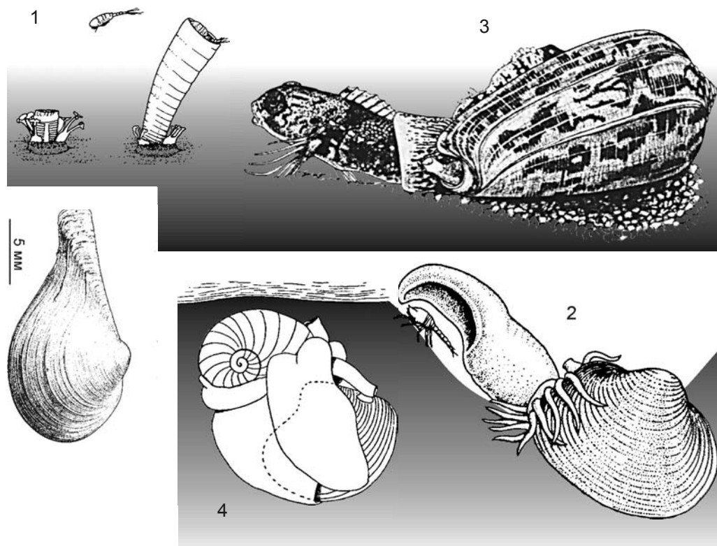
Рис. 2.20. Хищники.
