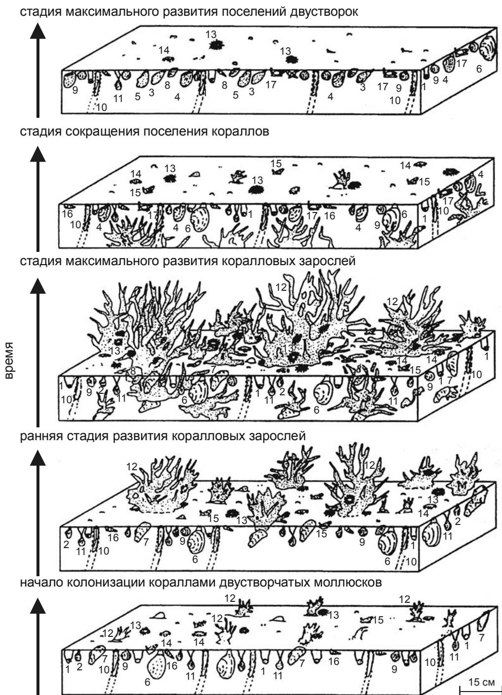
Рис. 3.53. Изменение состава сообществ при развитии поселений ветвистых кораллов на мелководье у атлантических берегов юга Северной Америки в плиоценовое время. По Bailey, Tedesco (1986) из Л.А. Невесской (1999: 330).
