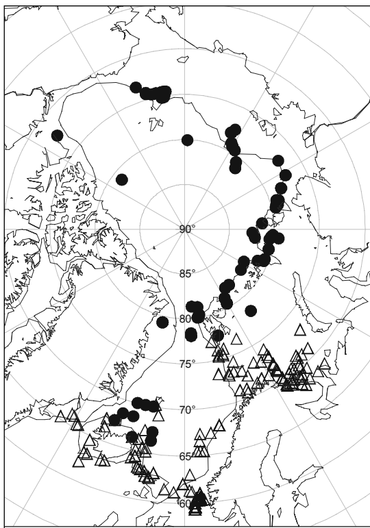
Рис. 6.17. Ареалы высокоарктических глубоководных видов (кружок): Melinnopsis arctica , Hyalopomatatus claparedii , Protis arctica , Paradiopatra pauli и комплементарное им в Северном Ледовитом океане распространение атлантических эврибатных видов (треугольник): Potamilla neglecta , Paramphinoe jeffreysii , Notoproctus oculus .
