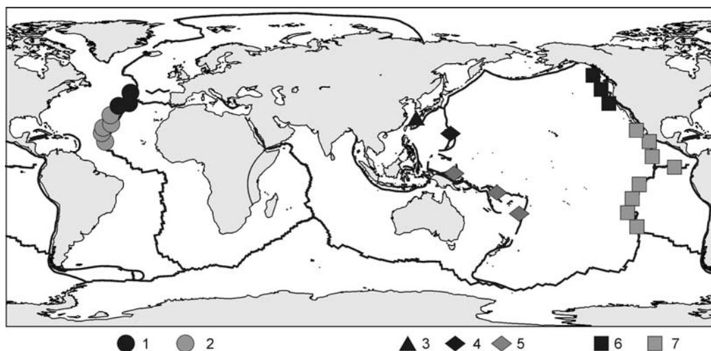
Рис. 3.75. Биогеографическое районирование гидротерм. По С.В. Галкину (2002).
