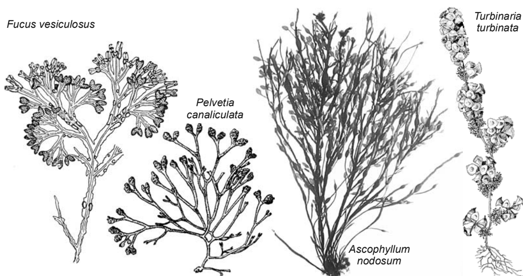
Рис. 3.31. Фукоиды.
