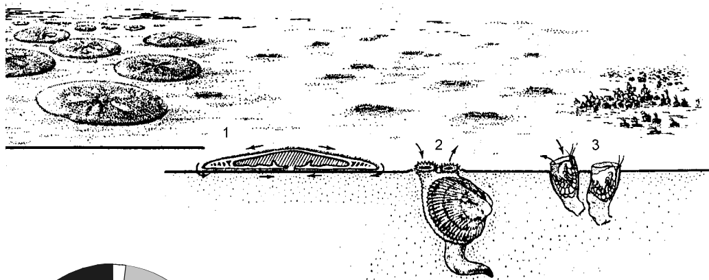
Рис. 3.12. Сообщество с доминированием фильтраторов инфауны. 1 — морские ежи Echinarachnius parma ; 2 — двустворчатые моллюски Ciliatocardium ciliatum ; 3 — бокоплавы Ampelisca . По А.И. Савилову (1961).
