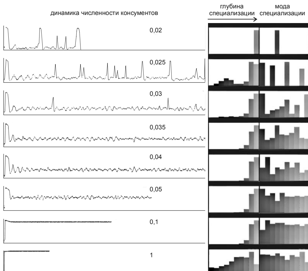
Рис. 4.40. Динамика численности консументов в зависимости от продуктивности.
