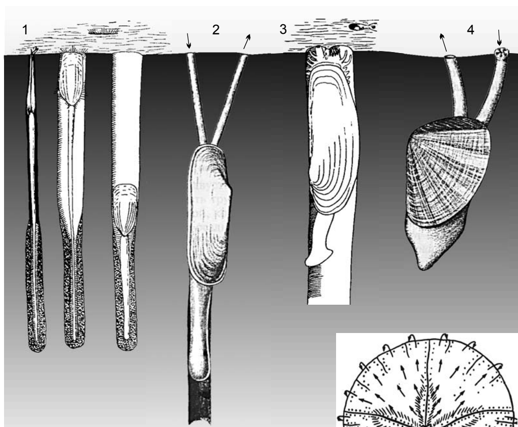
Рис. 2.15. Фильтраторы инфавны.
