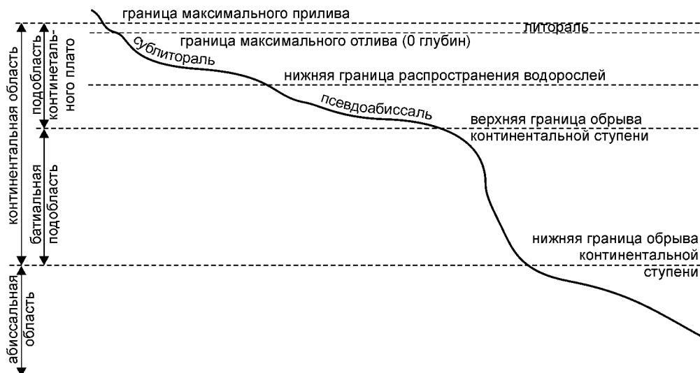
Рис. 6.1. «Схема морских зон» Комиссии 2-го Всесоюзного гидрологического съезда. По Аноним (1928) из А.П. Андрияшева (1979).
