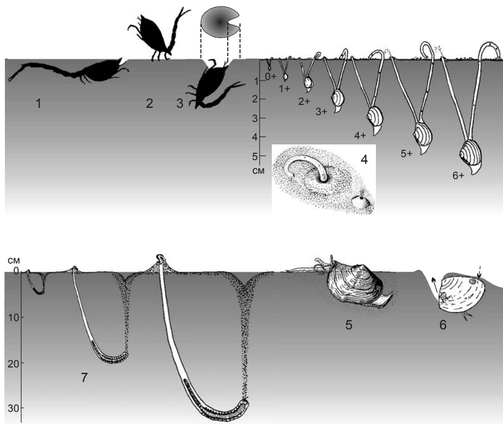
Рис. 2.17. Собирающие детритофаги.
