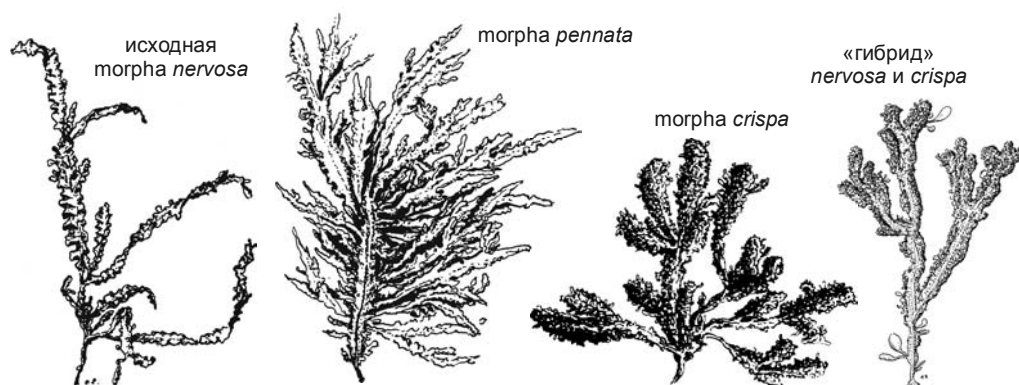
Рис. 3.52. Морфотипы прикреплённой Phyllophora nervosa . По О.В. Максимовой, П.В. Рыбникову (1993).
