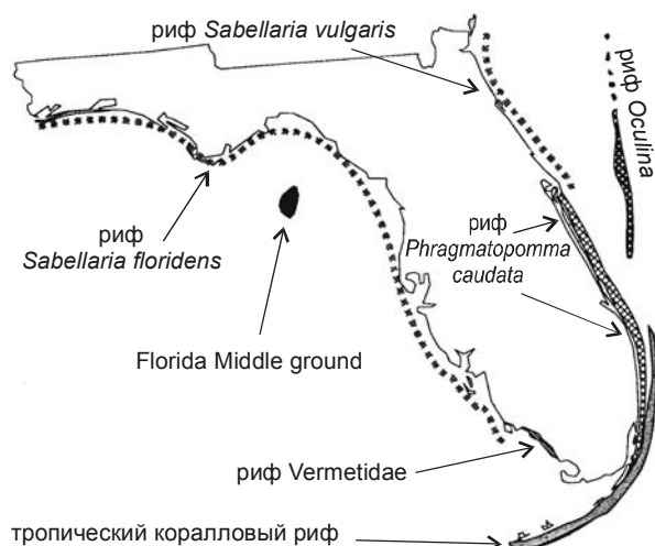
Рис. 3.55. Распределение рифов у берегов Флориды. По Perry (1992).
