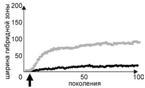
Рис. 4.34. Динамика ширины гибридной зоны при беспрепятственной гибридации и конкурентном исключении в зависимости от радиуса расселения. Стрелкой отмечен момент контакта, серая линия — большой радиус, черная — меньший.
