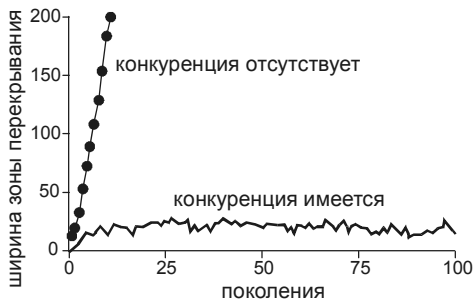
Рис. 4.33. Динамика ширины зоны перекрывания ареалов в отсутствии гибридации.
