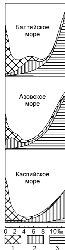
Рис. 1.22. Схема изменения числа видов по градиенту солёности в различных морях.
