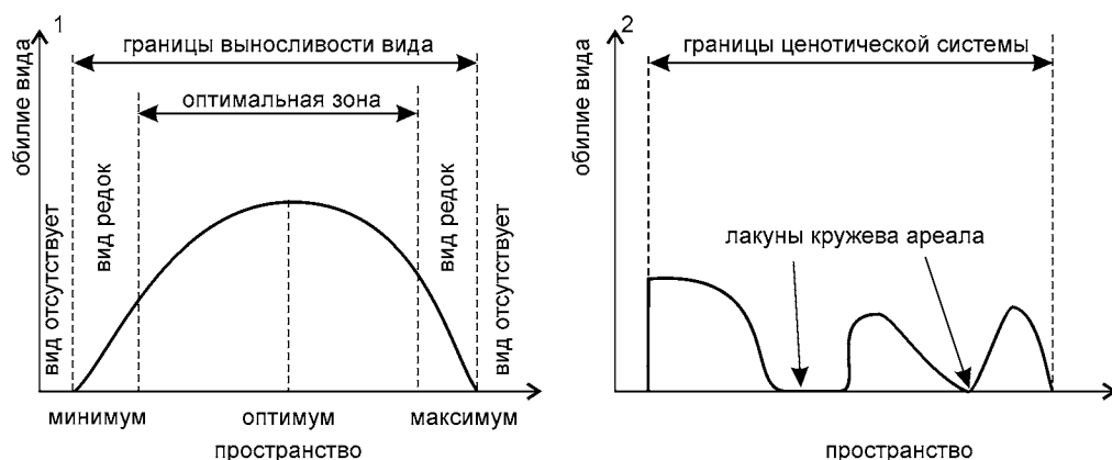
Рис. 5.10. Распределение обилия вида в пределах его ареала.
