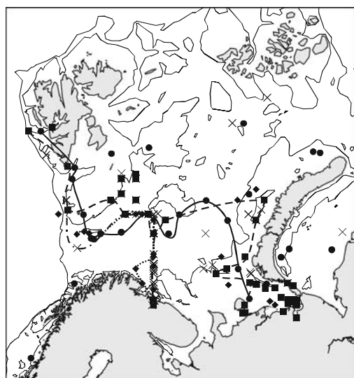
Рис. 5.19. Находки арктических шельфовых видов и границы их ареалов.
