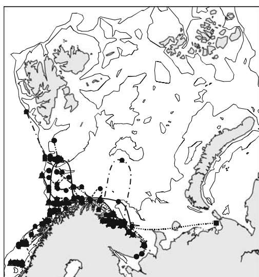
Рис. 5.20. То же, что и на рис. 5.19, но бореальных шельфовых видов.
