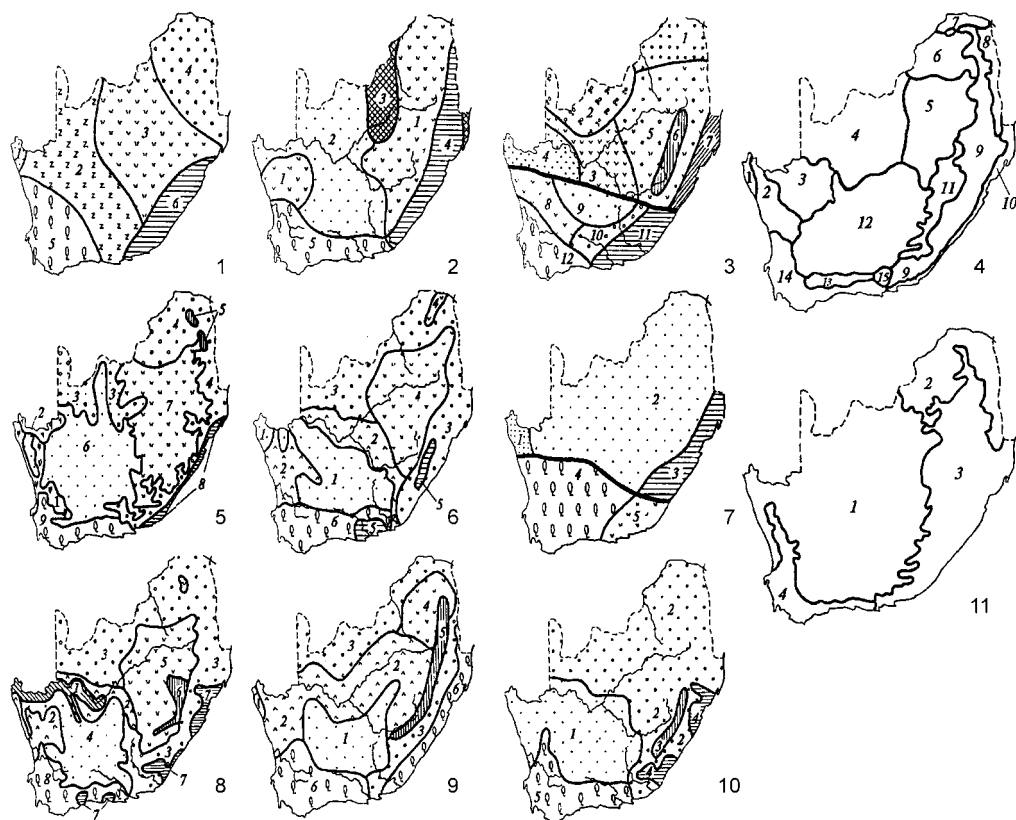
Рис. 5.12. Районирование Южной Африки по растительности.
