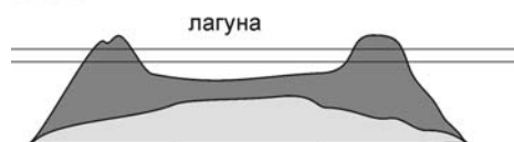
Рис. 3.61. Типы коралловых рифов.
