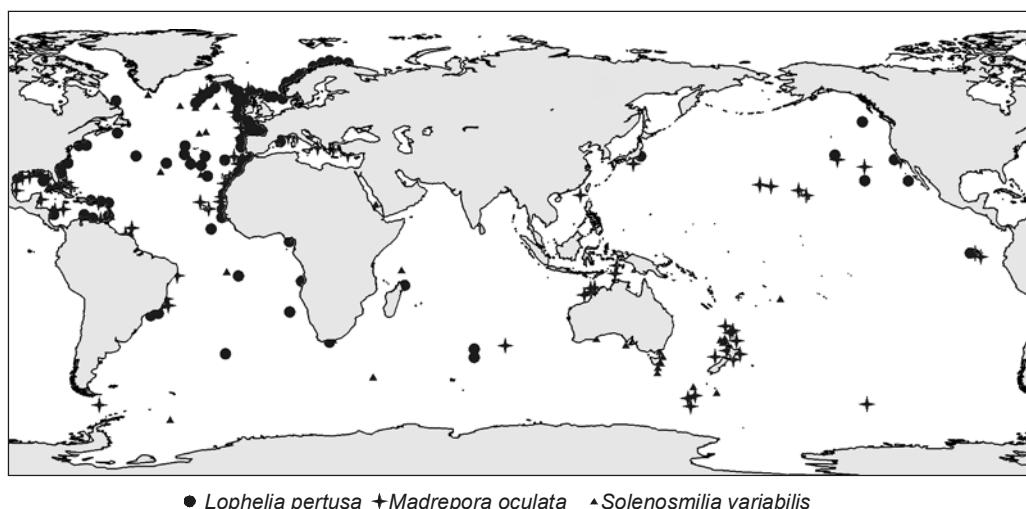
Рис. 3.70. Распространение глубоководных коралловых рифов.
