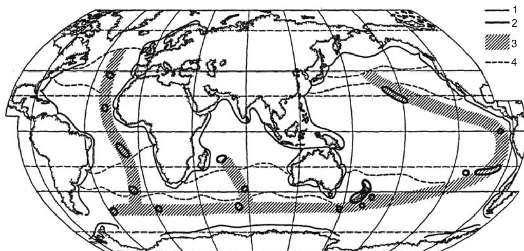
Рис. 6.13. Гипотетическая схема фаунистического районирования сублиторали и верхней батии Мирового океана А.Н. Миронова (1994).
