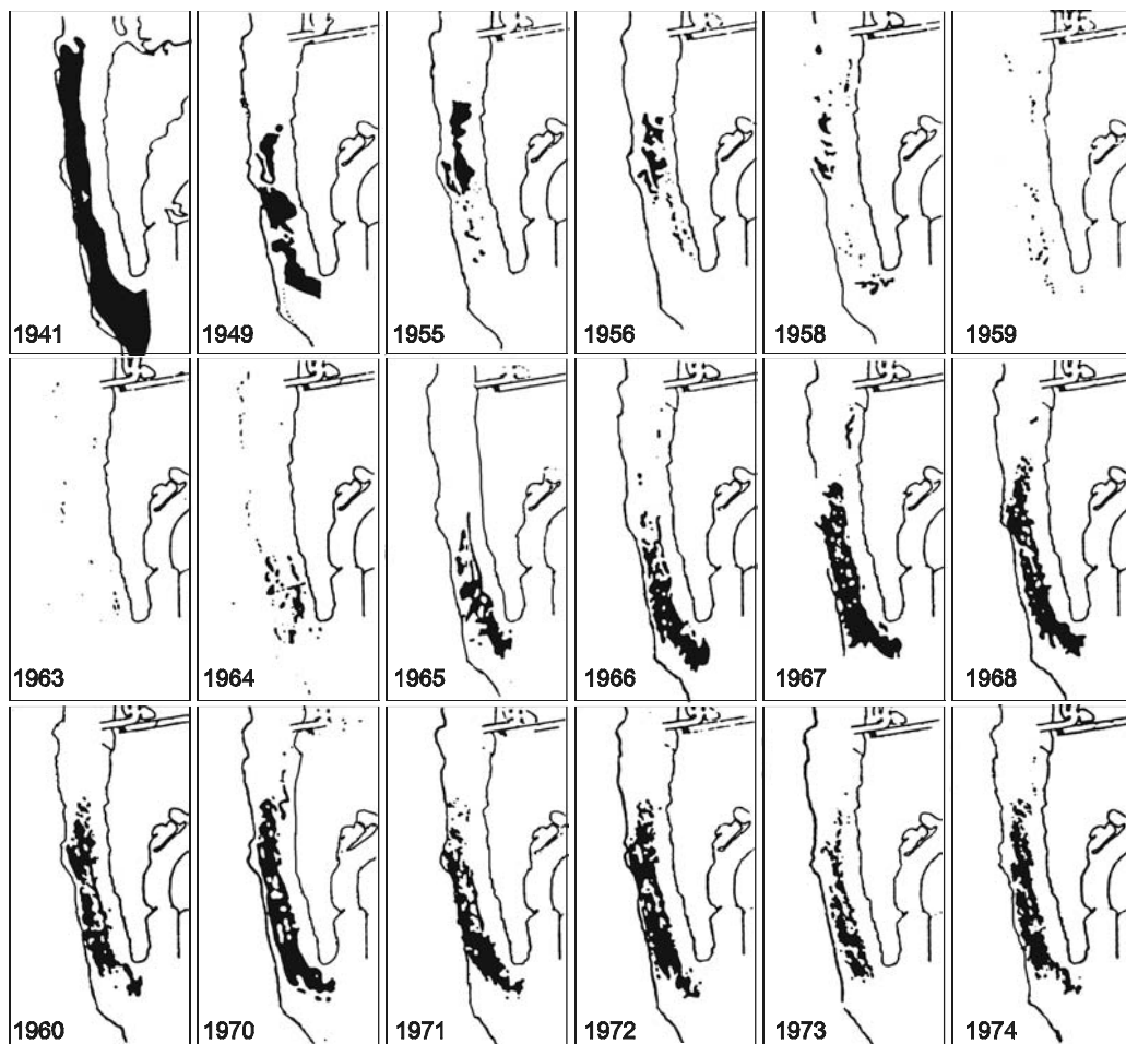
Рис. 3.41. Динамика келпов Macrocytis pyrifera у Point Loma, Калифорния.
