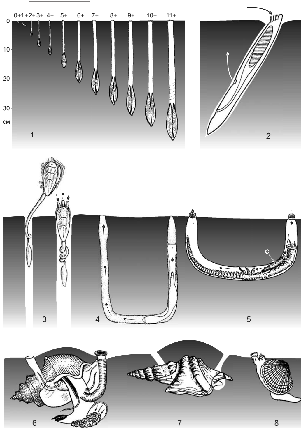
Рис. 2.14. Фильтраторы инфауны.
