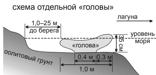
Рис. 3.37. Рифы багрянок в Тунисе. По Thornton et al. (1978).
