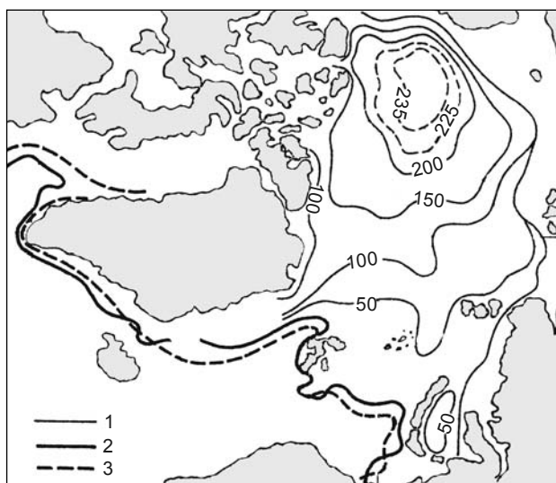
Рис. 1.19. Распреснённая линза.
