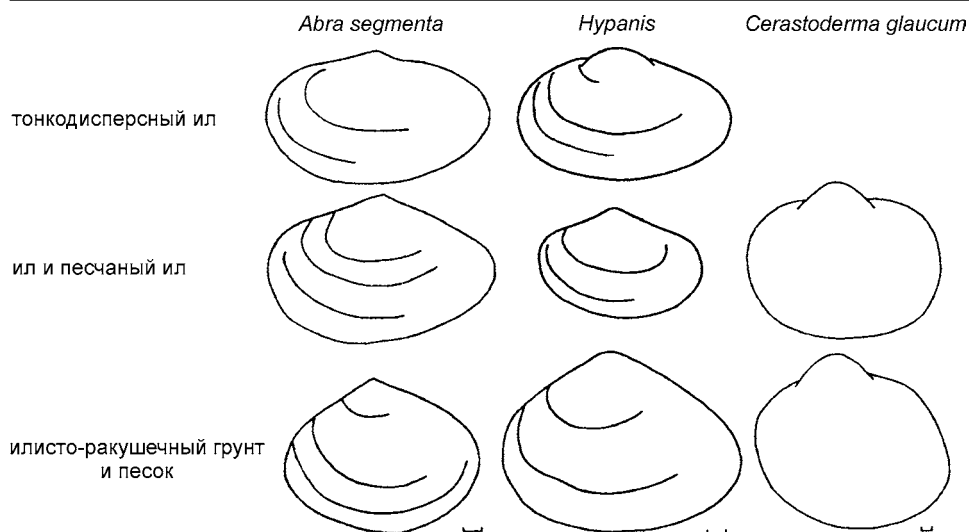
Рис. 4.20. Жизненные формы инфаунных двусторчатых моллюсков Арала. По С.И. Андреевой (2001).
