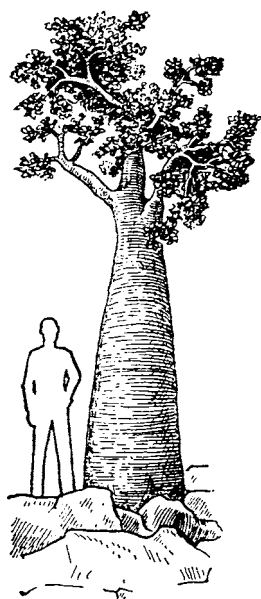
Рис. 4.14. Dendrosicyos socotranus . По Денисовой (1981).
