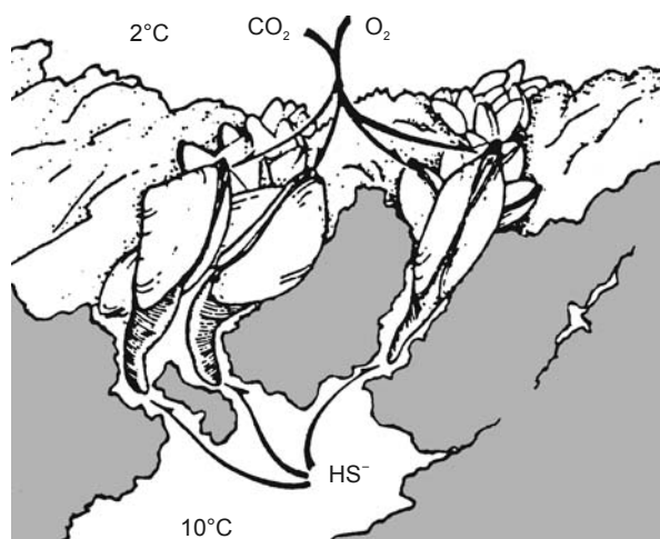
Рис. 2.7. Схема расположения Calyptogeno magnifica в грунте. По Arp et al. (1984).
