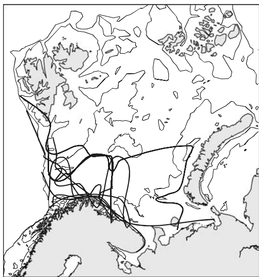
Рис. 5.21. Ступение границ ареалов.
