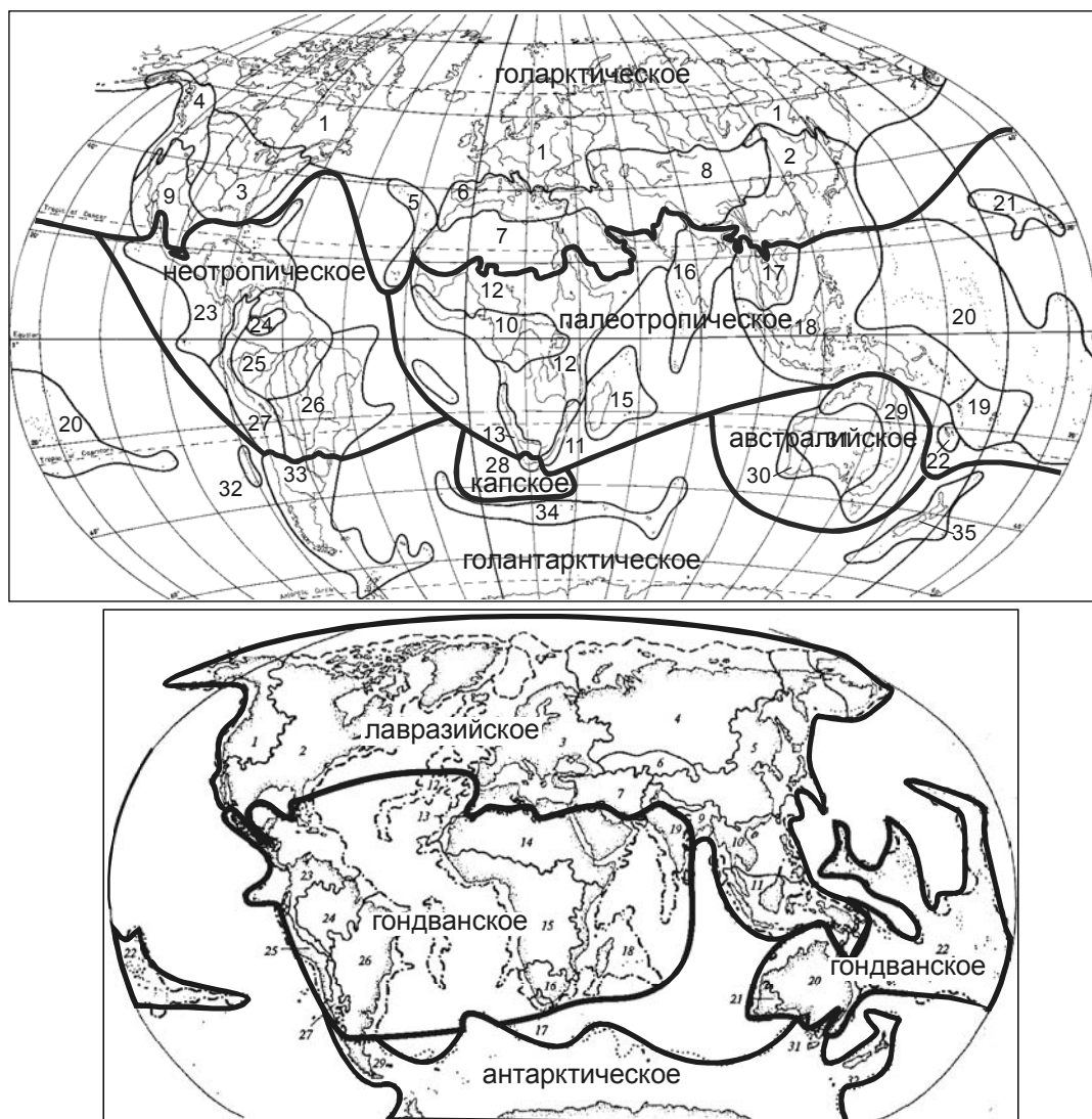
Рис. 5.14. Различные схемы фитогеографического районирования суши: сверху — А.Л. Тахтаджяна (1986, мало отличающиеся схемы опубликованы в 1974 и 1978), внизу — С.М. Разумовского (1999).
