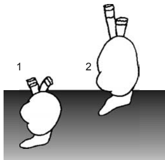
Рис. 4.19. Разные экотипы Cerastoderma Аральского моря. По С.И. Андреевой (2001).
