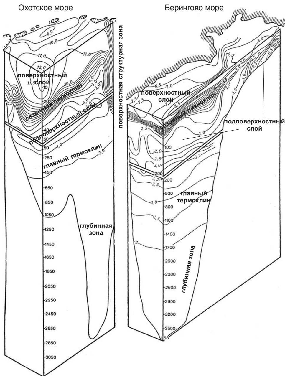
Рис. 1.8. Примеры распределения температуры по глубине. По А.Д. Добровольскому, Б.С. Залогину (1982).
