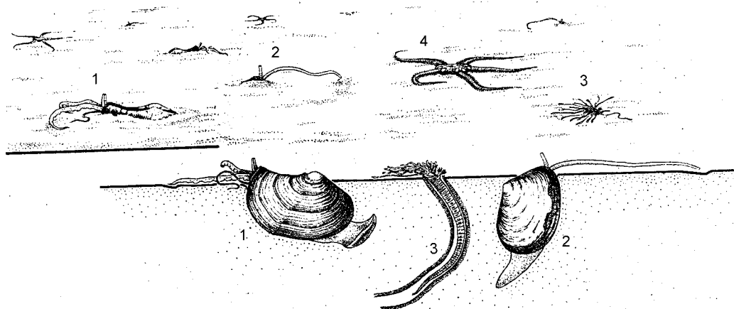
Рис. 3.14. Сообщество с доминированием собирающих детритофагов. Двустворчатые моллюски: 1 — Yoldia thracieformis и 2 — Macoma calcarea ; 3 — полихеты Terebellidae ; 4 — офиуры Ophiura sarsi . По А.И. Савилову (1961).
