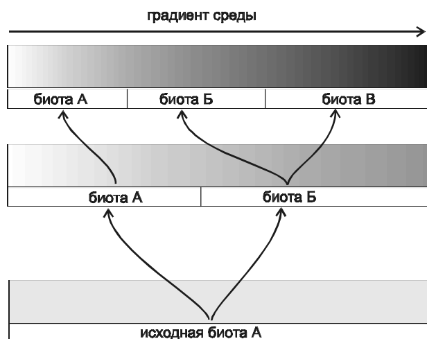
Рис. 4.26. Возникновение видов и биот с позиции структуризма.
