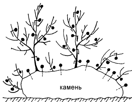
Рис. 3.50. Схема эксперимента с гипсовыми шариками на цистозире (по: Хайлов и др., 1992).
