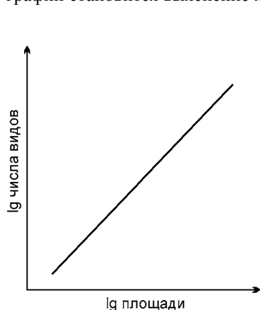
Рис. 5.30. Связь числа видов с площадью острова согласно теории островной биогеографии.
