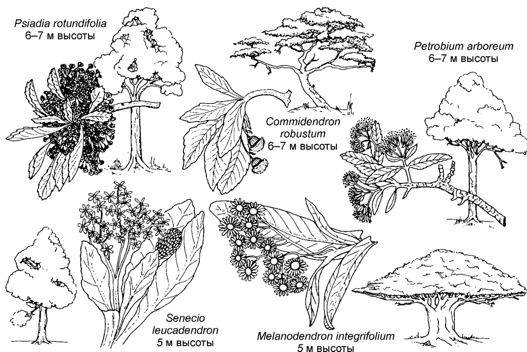
Рис. 4.13. Сложноцветные деревья о-ва Святой Елены. По Cox, Moore (2000).
