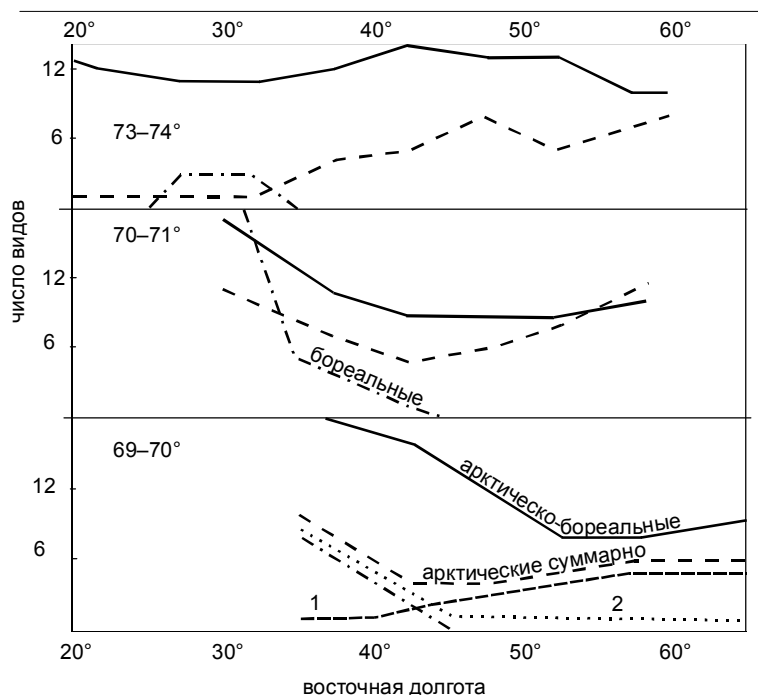
Рис. 5.18. Использование метода А.А. Шорыгина. 1 — арктические мелководные; 2 — арктические глубоководные виды. По А.А. Шорыгину (1928).
