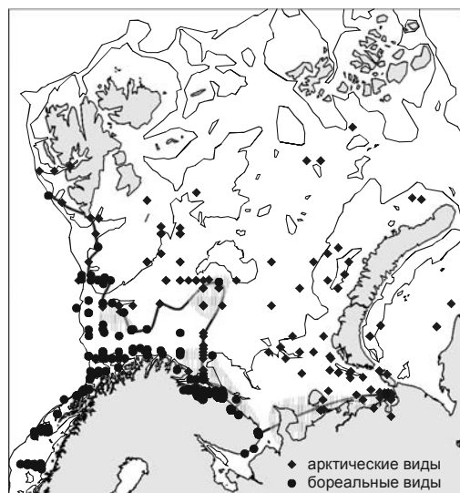
Рис. 5.22. Синперата. Заштрихованы области перекрывания ареалов.
