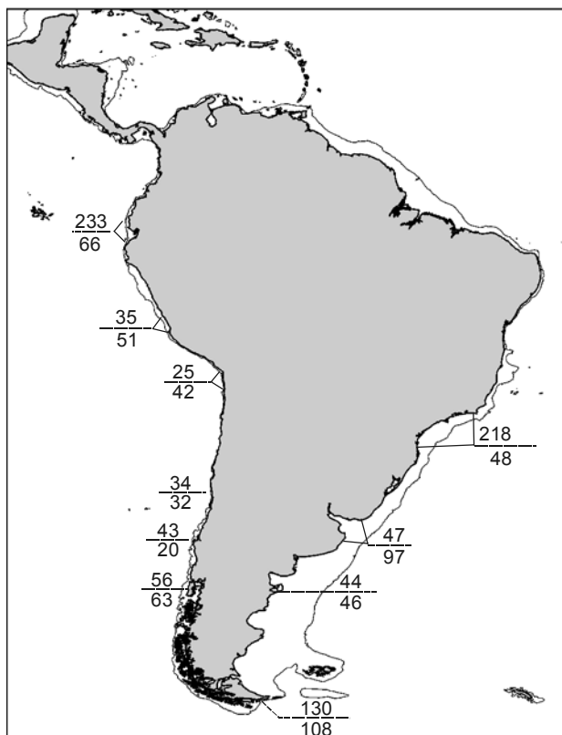
Рис. 5.29. Пример использования метода значимости биогеографических границ. По В.Н. Семёнову (1982).
