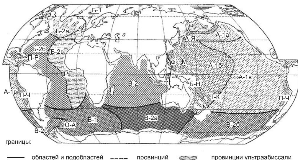
Рис. 6.14. Районирование абиссали и ультраабиссали Мирового океана Н.Г. Виноградовой (1977). А — тихоокеанско-североиндийская глубоководная область: А-1 — тихоокеанская подобласть (А-1а — северо-тихоокеанская, А-1б — западнотихоокеанская, А-1в — восточнотихоокеанская провинции); А-2 — североиндийская подобласть; Б — атлантическая глубоководная область: Б-1 — арктическая подобласть, Б-2 — атлантическая подобласть (провинции: Б-2а — североатлантическая, Б-2б — западноатлантическая, Б-2в — восточноатлантическая); В — антарктическая глубоководная область: В-1 — антарктическо-атлантическая подобласть, В-2 — антарктическо-индийско-тихоокеанская подобласть (провинции: В-2а — индийская, В-2б — тихоокеанская). Ультраабиссальные провинции: А-Я — алеутско-японская, Ф — филиппинская, М — марианская, Б-Н — бутенвильско-новогбридская, Т-К — тонго-кермадекская, П-Ч — перуано-чилийская, Я — яванская, П-Р — пуэрториканская, Р — жёлоба Романш, Ю-А — южноатлантическая.
