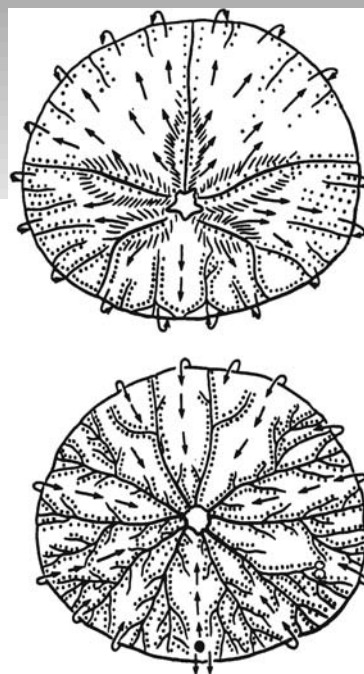
Рис. 2.16. Фильтраторы инфавны. Плоский морской еж Dendraster excentricus сверху и снизу.
