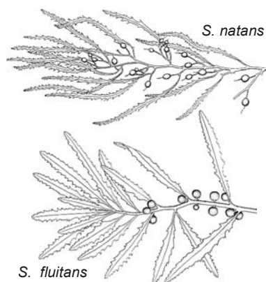
Рис. 3.38. Саргассы ( Sargassum ) Саргассова моря. По Taylor (1960).
