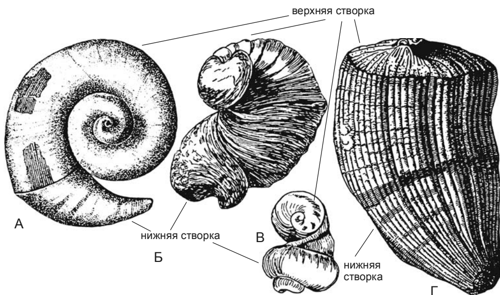
Рис. 3.67. Рудисты.
