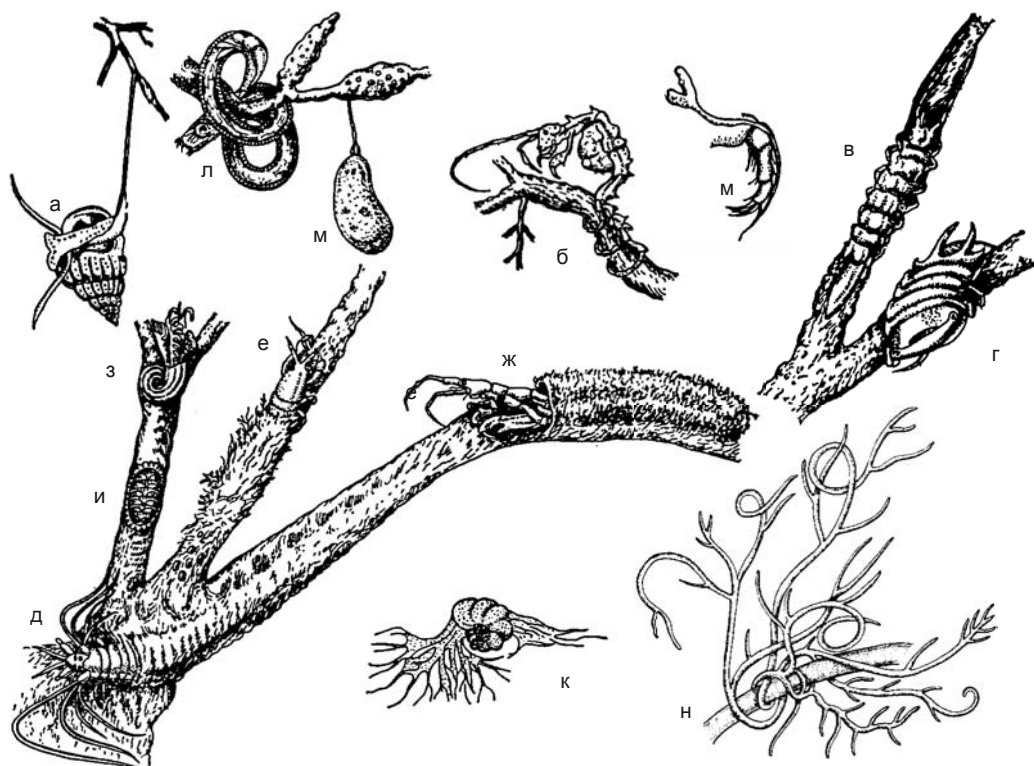
Рис. 3.27. Способы прикрепления эпифитона к макрофитам.
