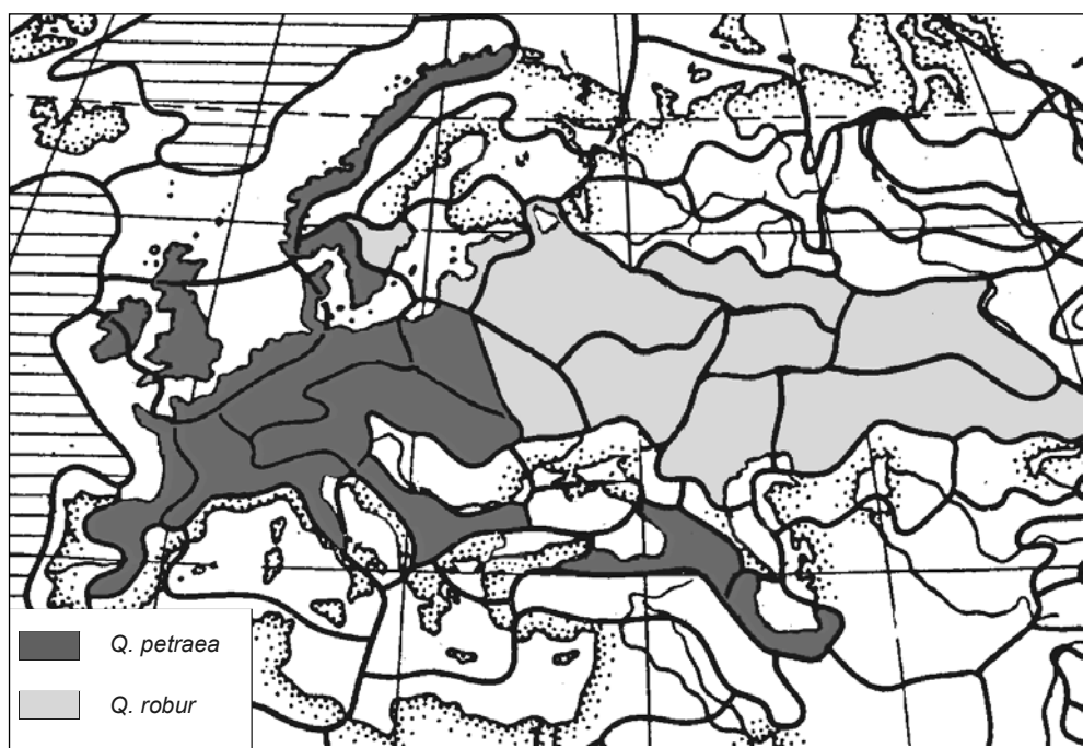
Рис. 4.38. ЦС, в которых эдификаторами климкса являются Quercus petraea и Q. robur . По С.М. Разумовскому (1999).
