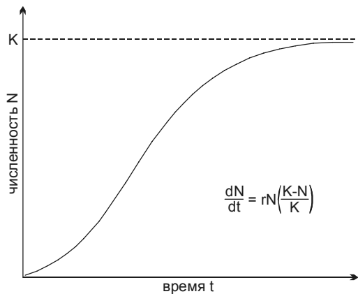
Рис. 2.22. Логистическая кривая роста численности популяции.
