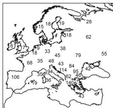
Рис. 5.36. Центры разнообразия покрытосемянных рода смолевка Silene . По Thompson (1973).
