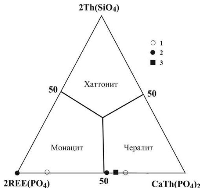
Рис. 6. Положение точек чералита из спессартин-кварцевых пород Сихотэ-Алиня на классификационной диаграмме 2\text{REE}(\text{PO}_4) - \text{CaTh}(\text{PO}_4)_2 - 2\text{Th}(\text{SiO}_4) (Linhout, 2007).
