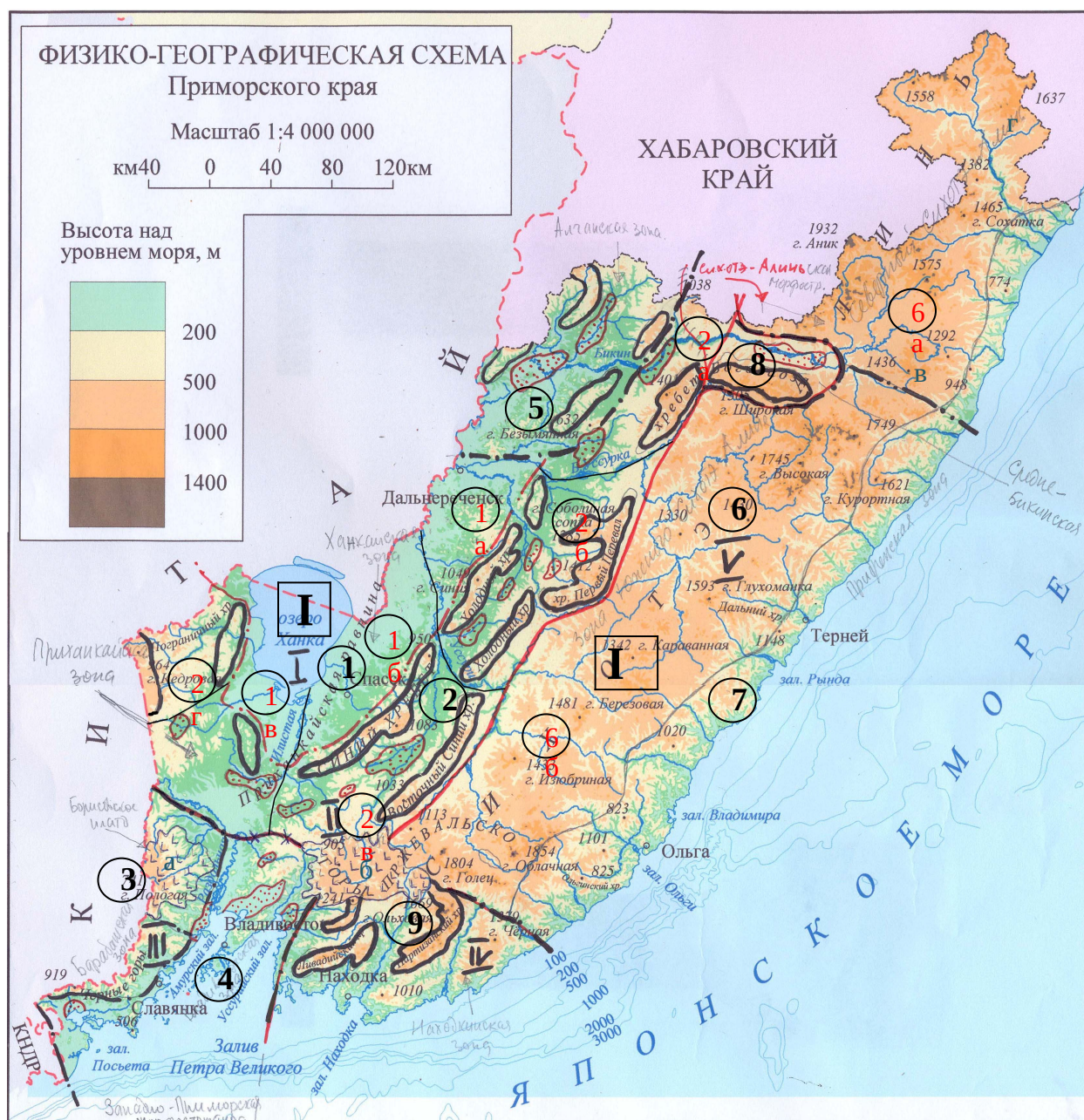
Рис. 1.1. Морфоструктурная схема Приморского края
